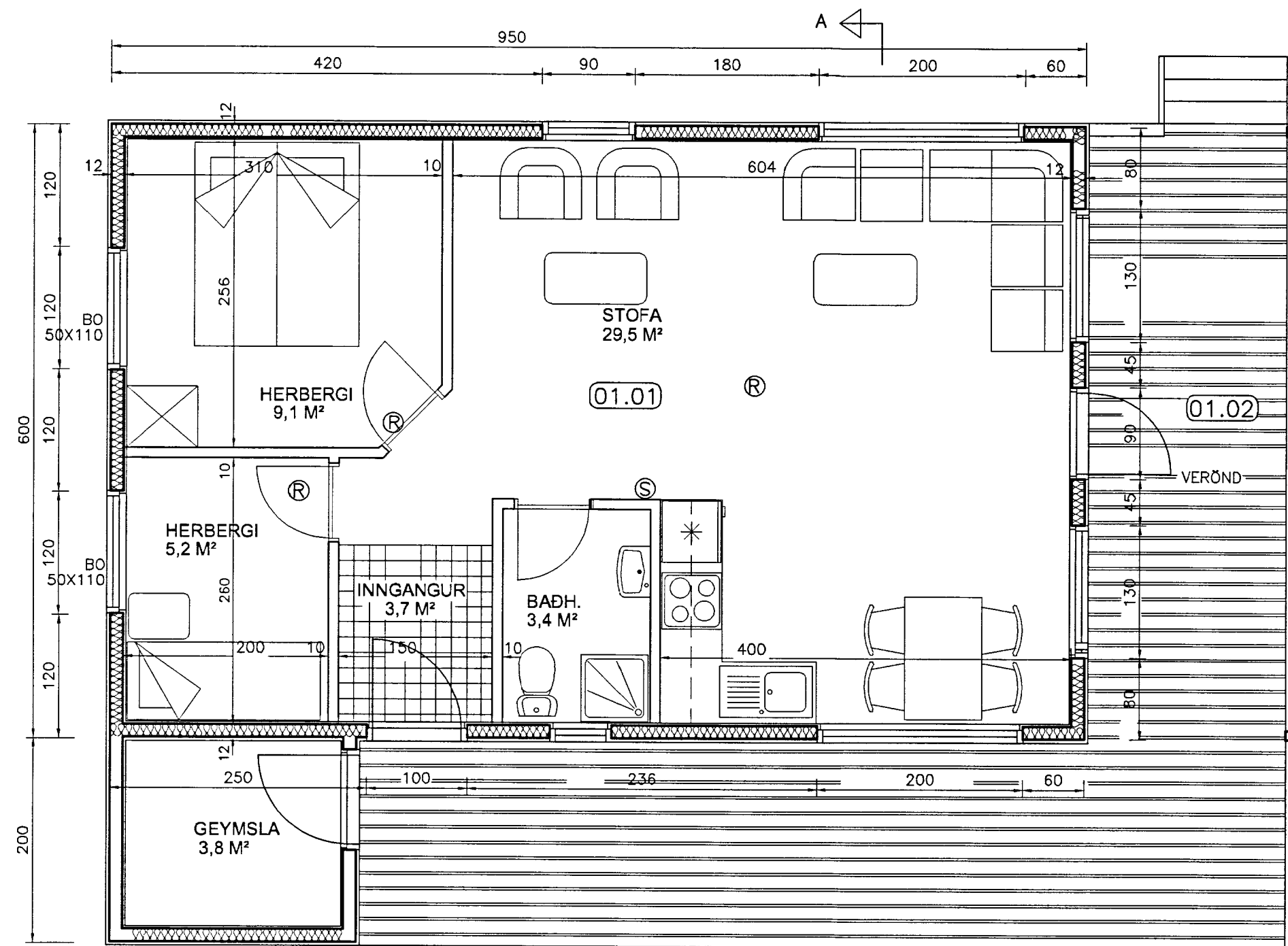
Grunnmynd mkv. 1:50
