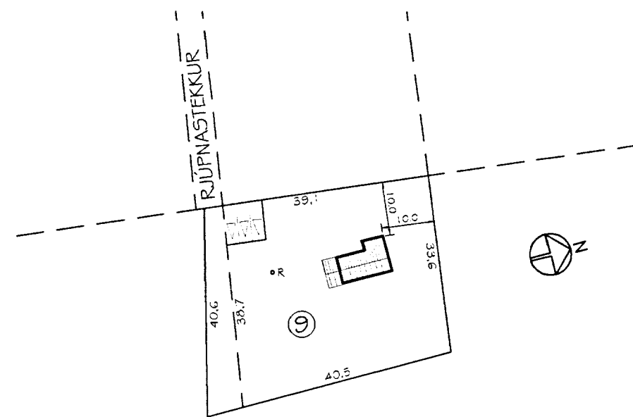
AFSTÖÐUMYND Mkv. 1:1000
