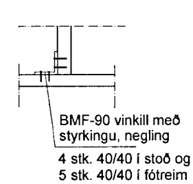
DEILI - C 1:20
