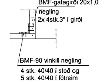
DEILI - E 1:20
