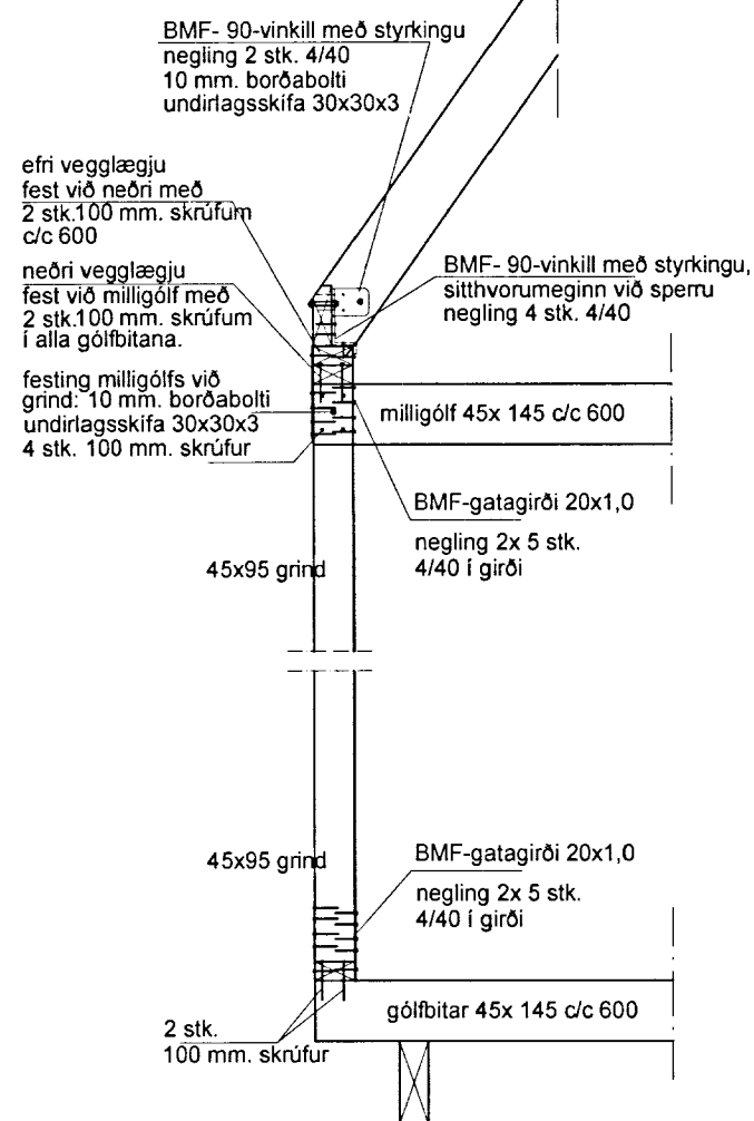
SNÍÐ C-C 1:20
