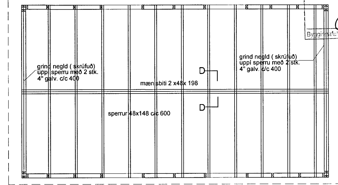
Grunnmynd 1:50 Þakviðir
