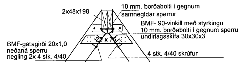
SNÍÐ D-D 1:20
