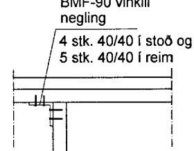
DEILI - B 1:20
