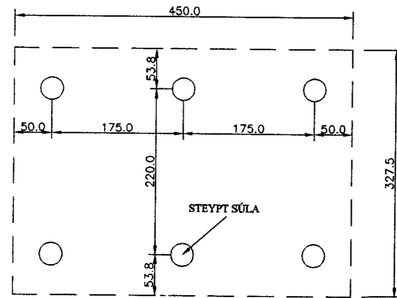
Grunnmynd steypar súlur
