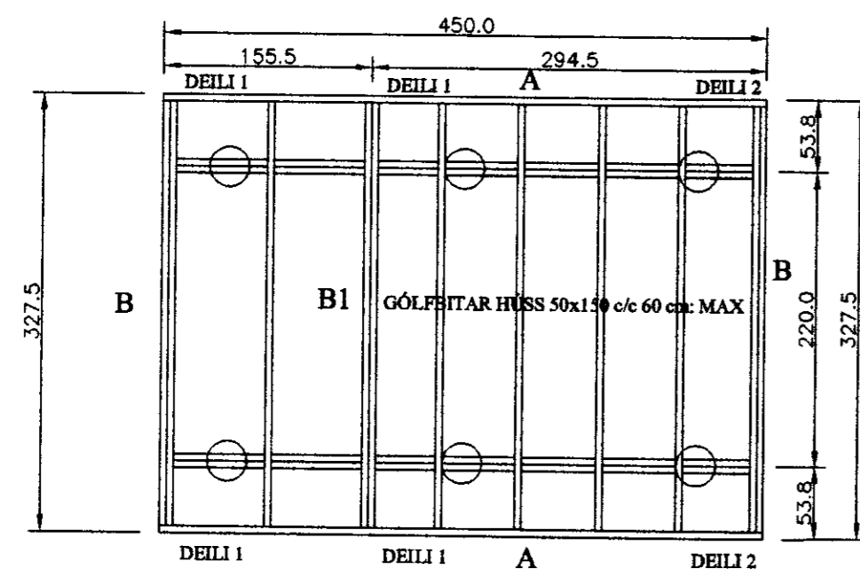
Grunnmynd gólfbitar
