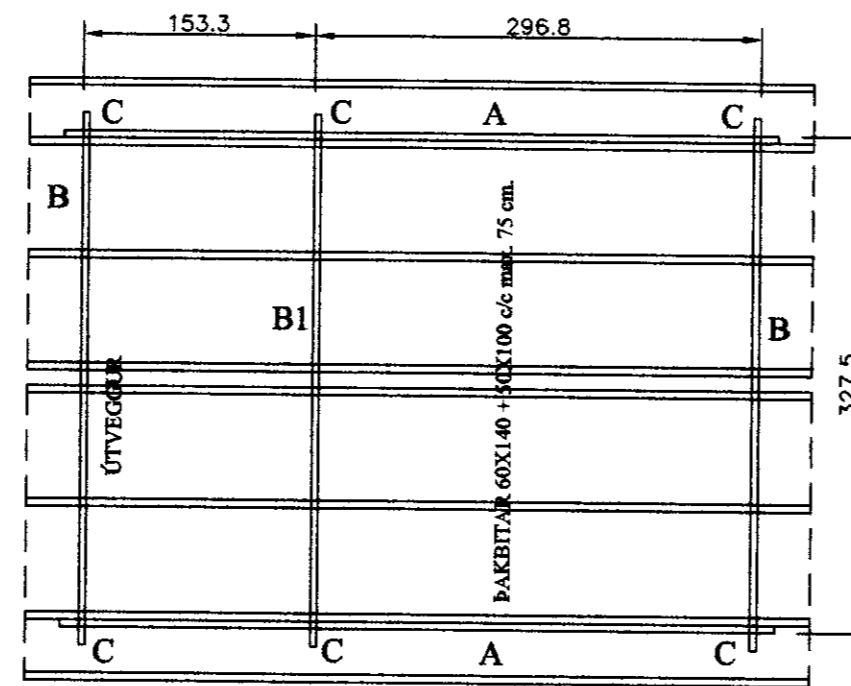
Grunnmynd þak
