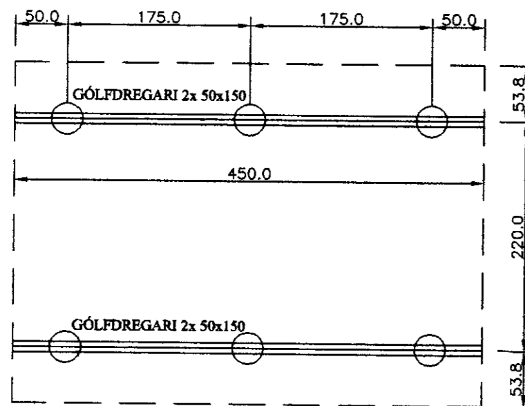
Grunnmynd dregarar
