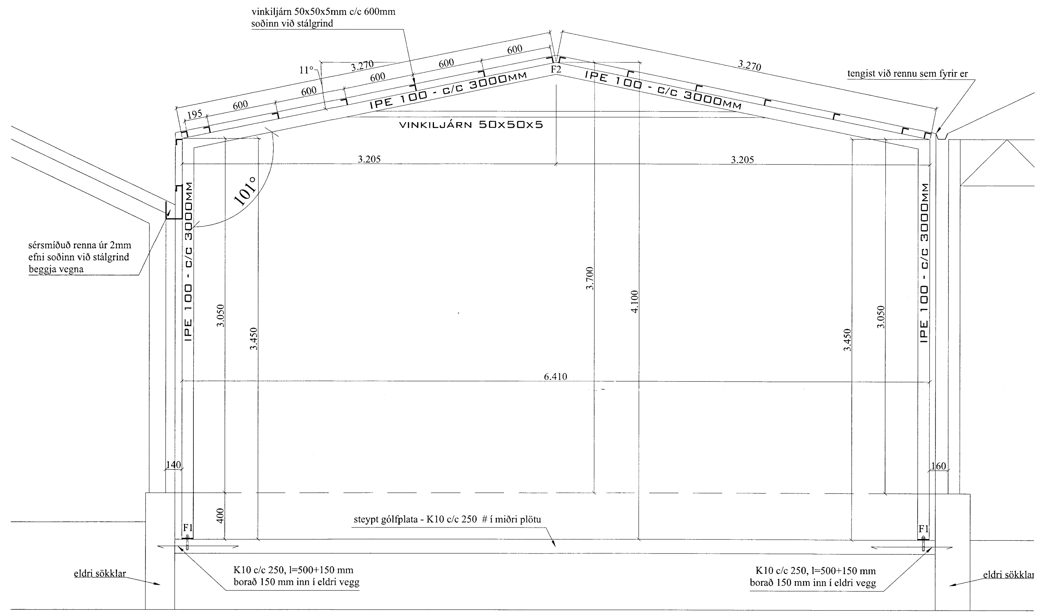
SNID A-A MKV. 1:20
