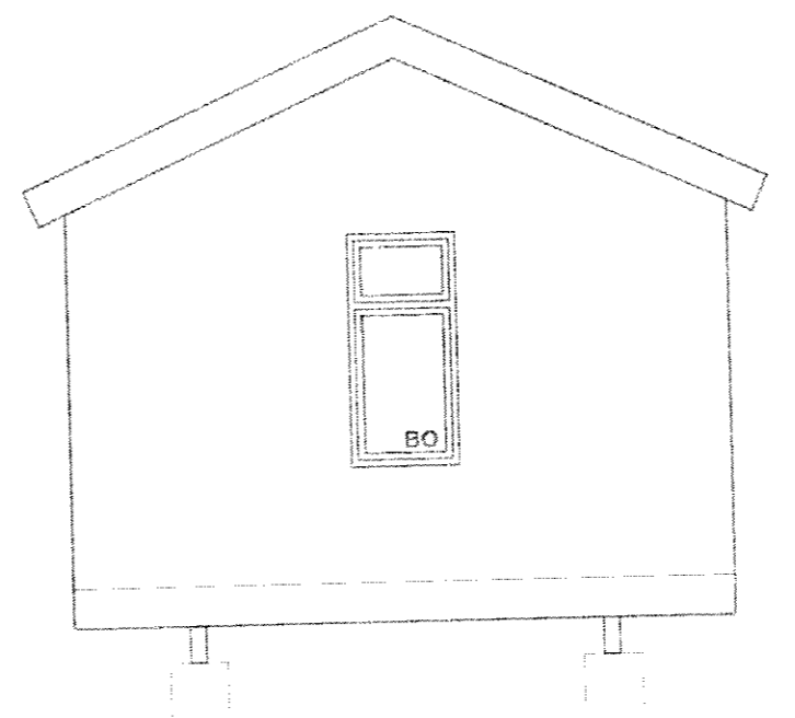
ÚTLIT - NORDUR
