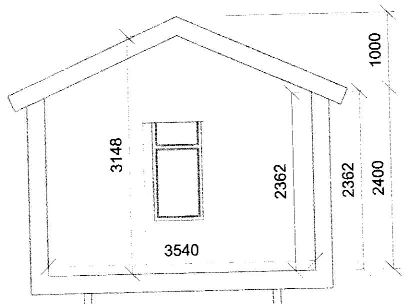
ÚTLIT - NORDUR
