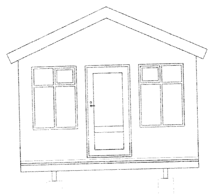
ÚTLIT - SUÐUR
