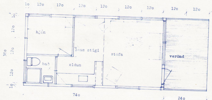
GRUNNMYND 1:50
