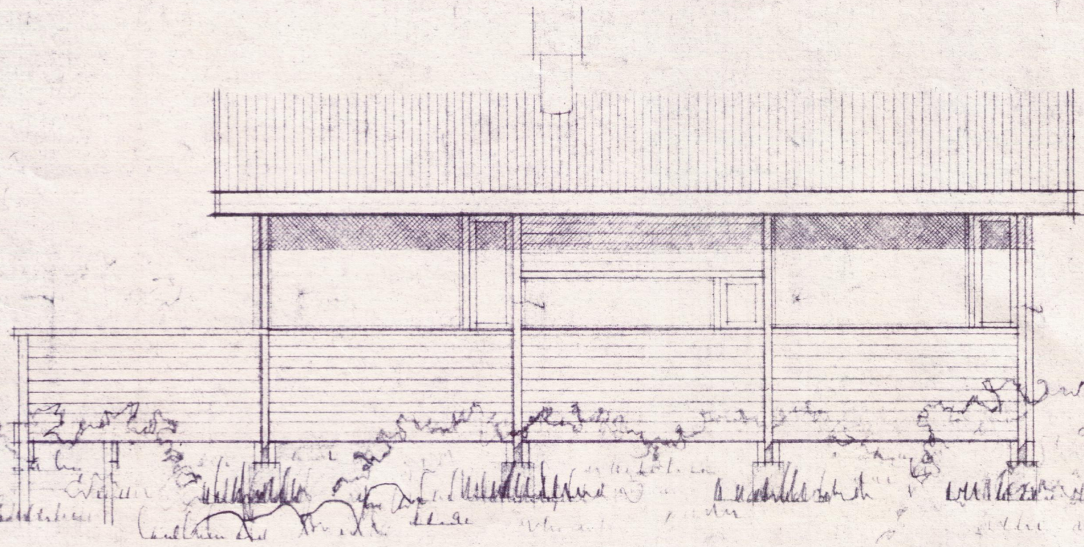
AUSTURHLID
