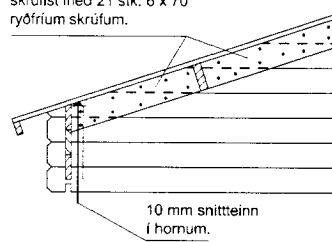
STYRKING Í GAFLI 1 : 20
