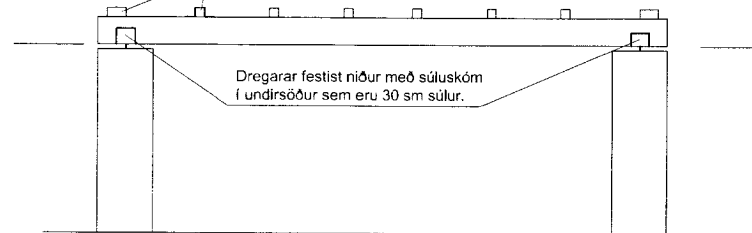
SNIÐ A - A 1 : 20
