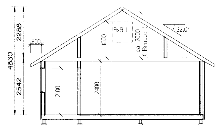
SNIÐ A-A MKV. 1:100
