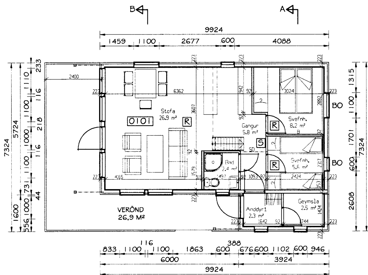
GRUNNMYND NEÐRI HÆÐAR MKV. 1:50
