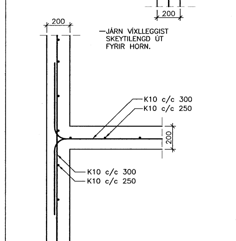
LÁRÉTT SNID Í SÖKKULVEGG Mkv. 1:20
