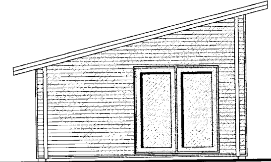
Suður M= 1:100
