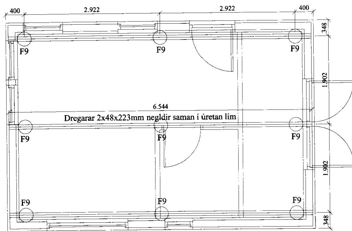
Grunnmynd súlna og dregara mkv. 1:50
