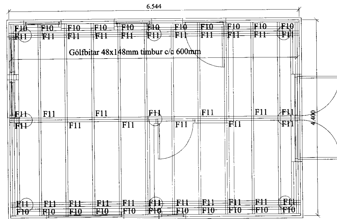
Grunnmynd gólfbita mkv. 1:50
