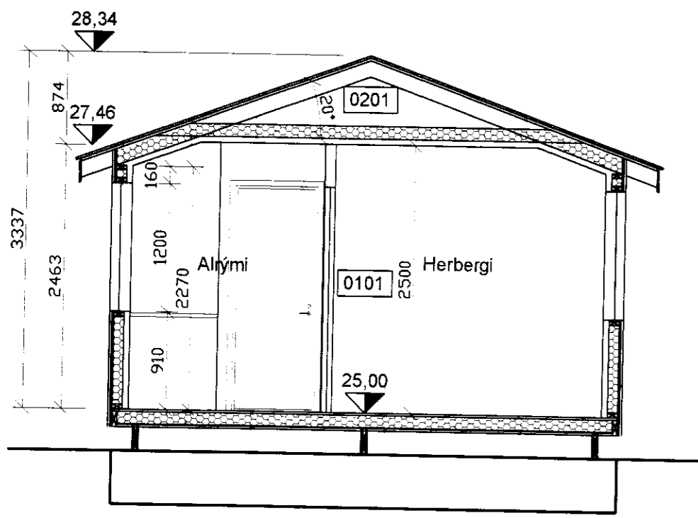
○ Snið A - 1:50
