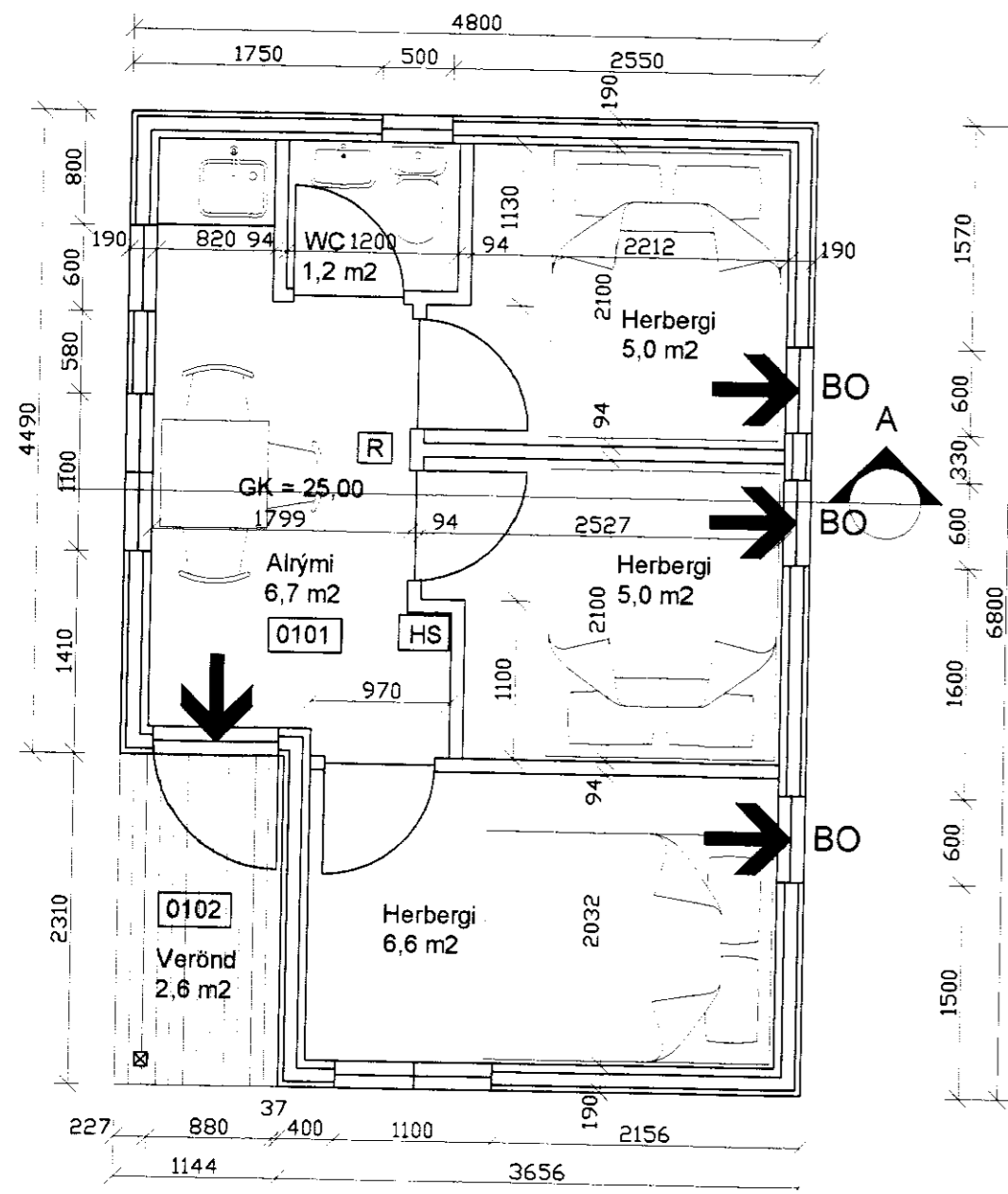
○ Grunnmynd - 1:50
