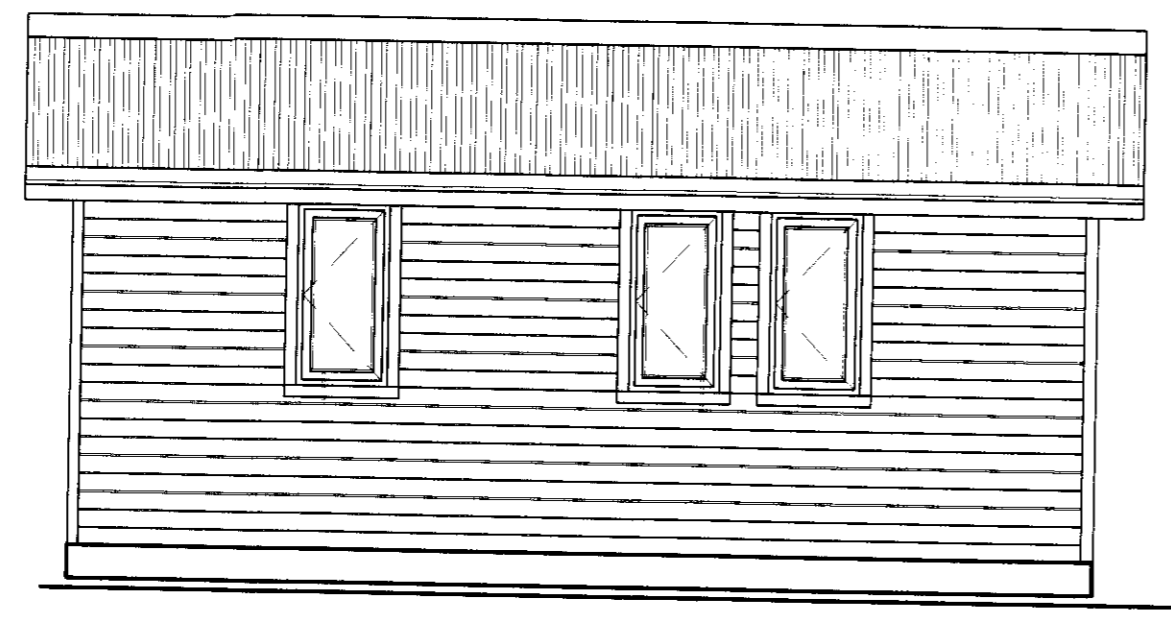
○ Suðurhlið - 1:50
