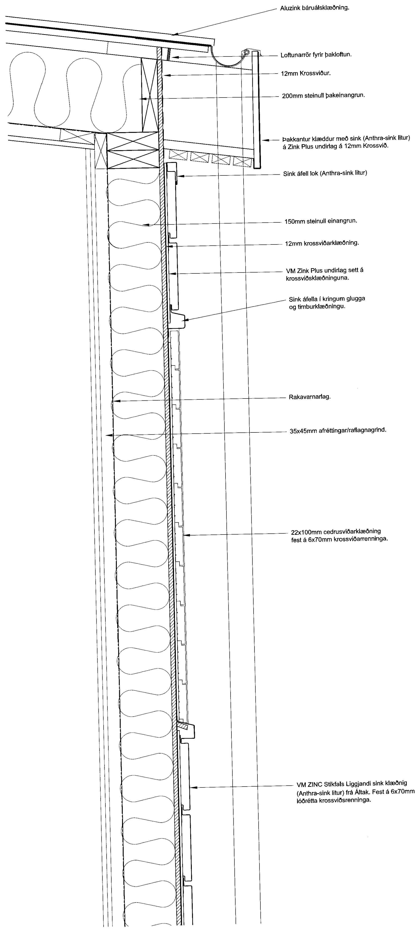
SNIDDEILI Í ÚTVEGG 1:5
