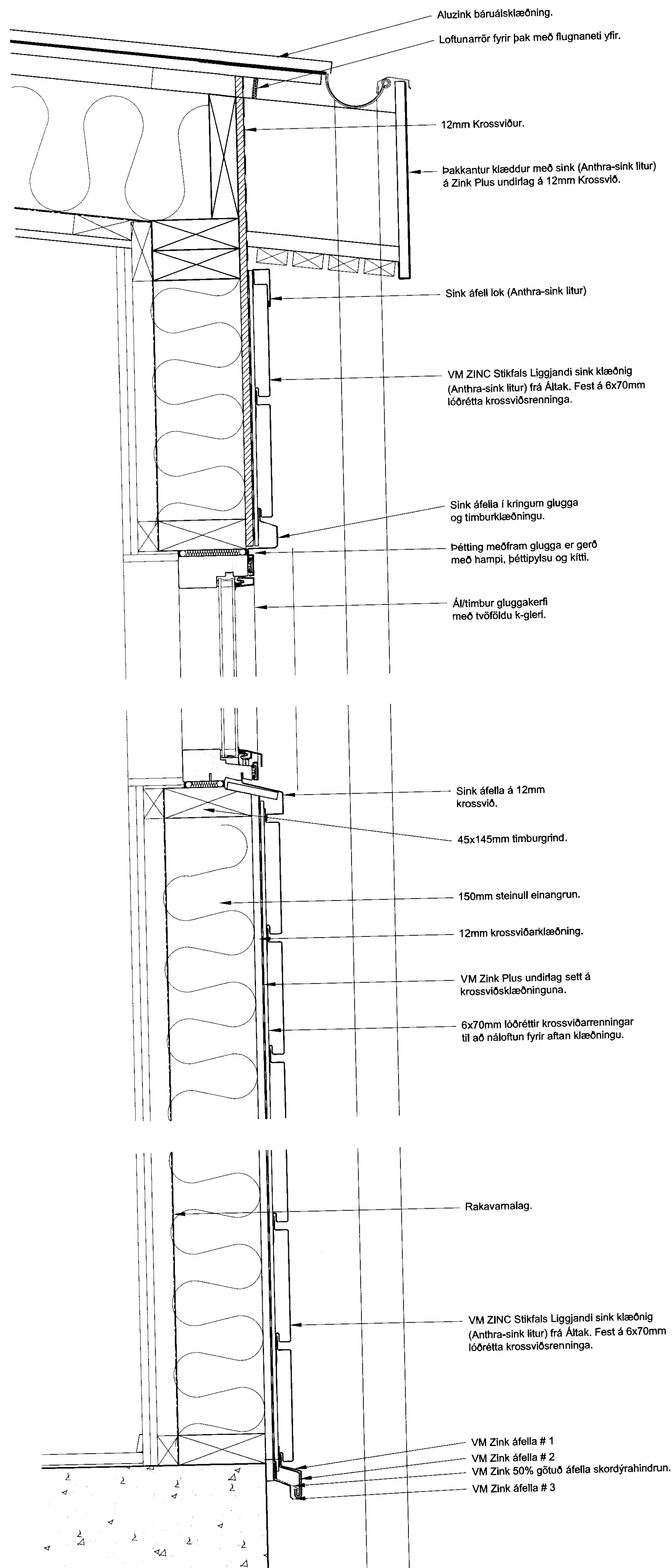
SNIDDEILI Í ÚTVEGG 1:5
