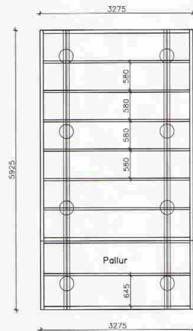
Grunnmynd dregarar
