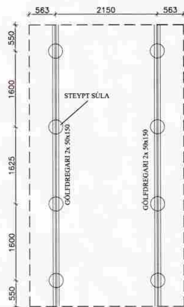
Grunnmynd steyptar súlur
