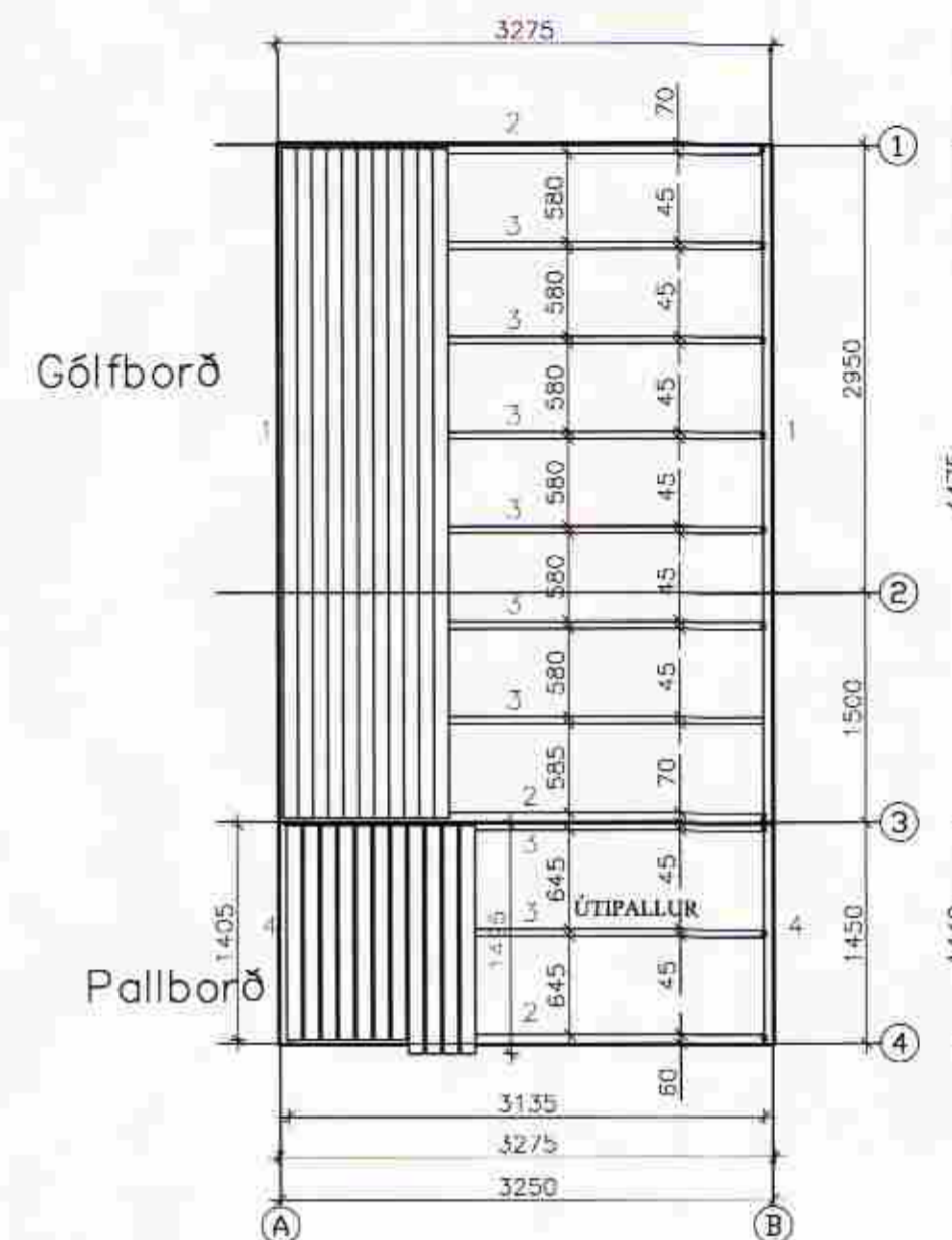
Grunnmynd gólfborð
