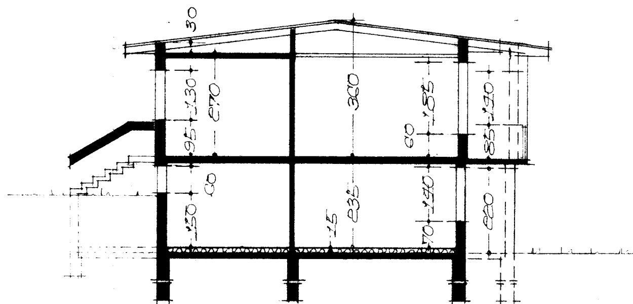
SKURÐUR A-A
