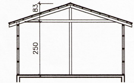
SNIÐ A-A
