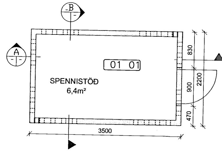
GRUNNMYND M 1:50
