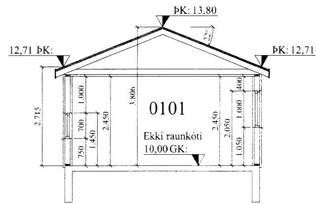
SNID A-A
