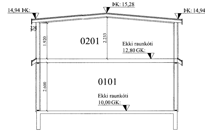
SNID D-D
