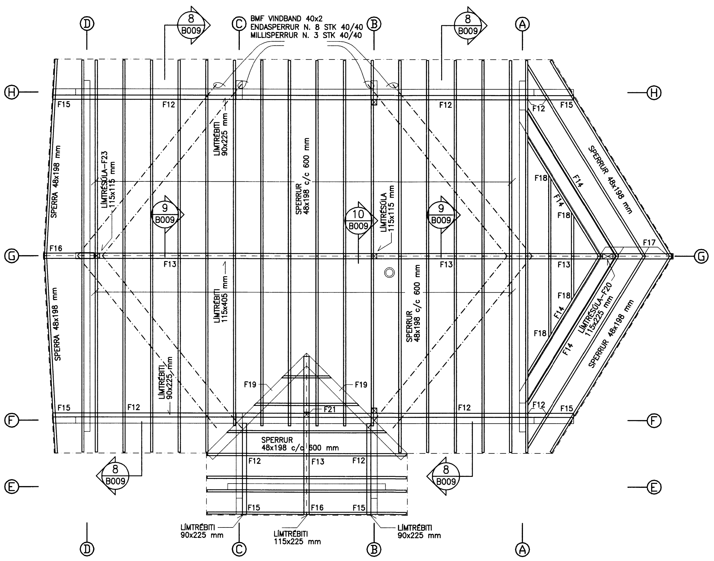
GRUNNMYNDR SPERRUPLAN 1:50
