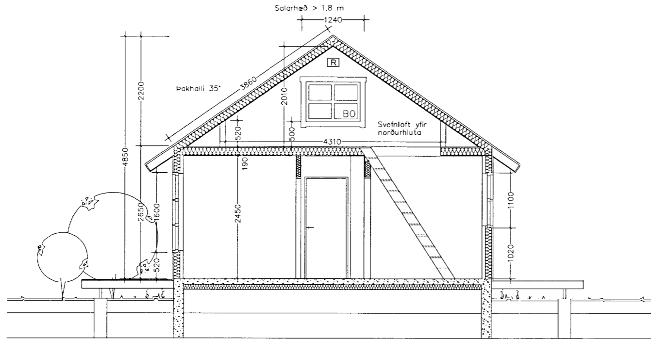
ÞVERSNIÐ
