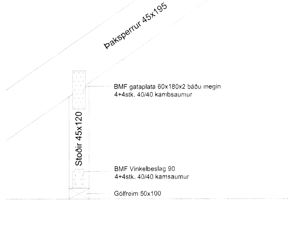
B-B Þakstólar millilofti
