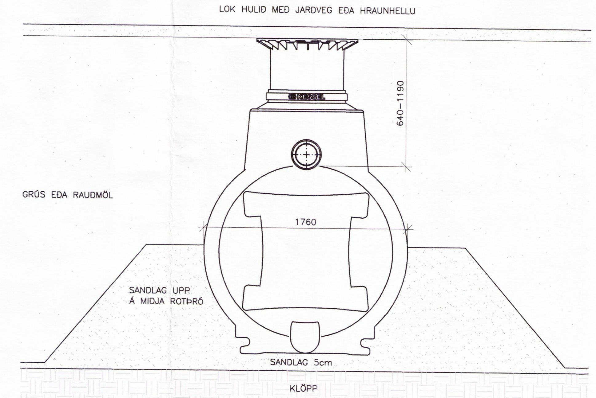
SNÍÐ Í SKÖLPHREINSISTÖÐ 1:20
