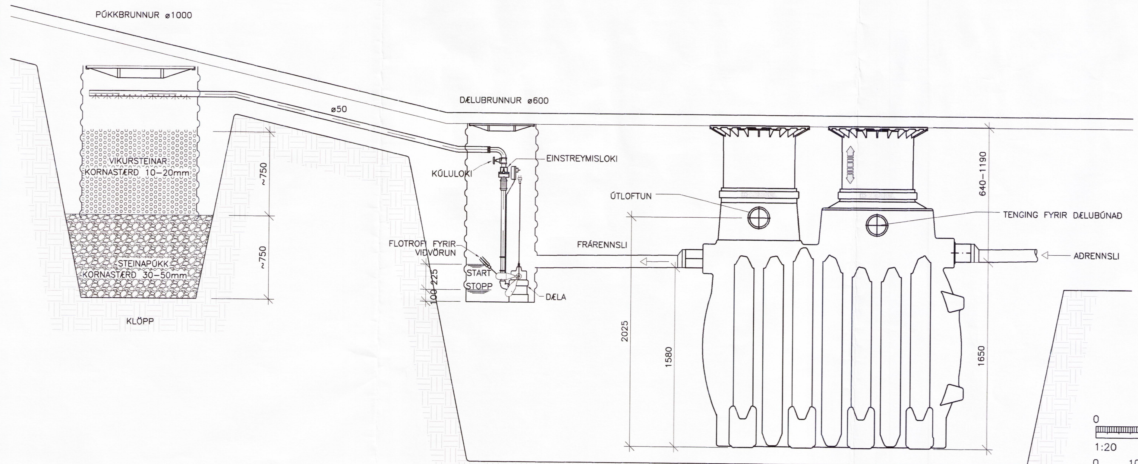
SNÍÐ Í SKÖLPHREINSISTÖÐ 1:20
