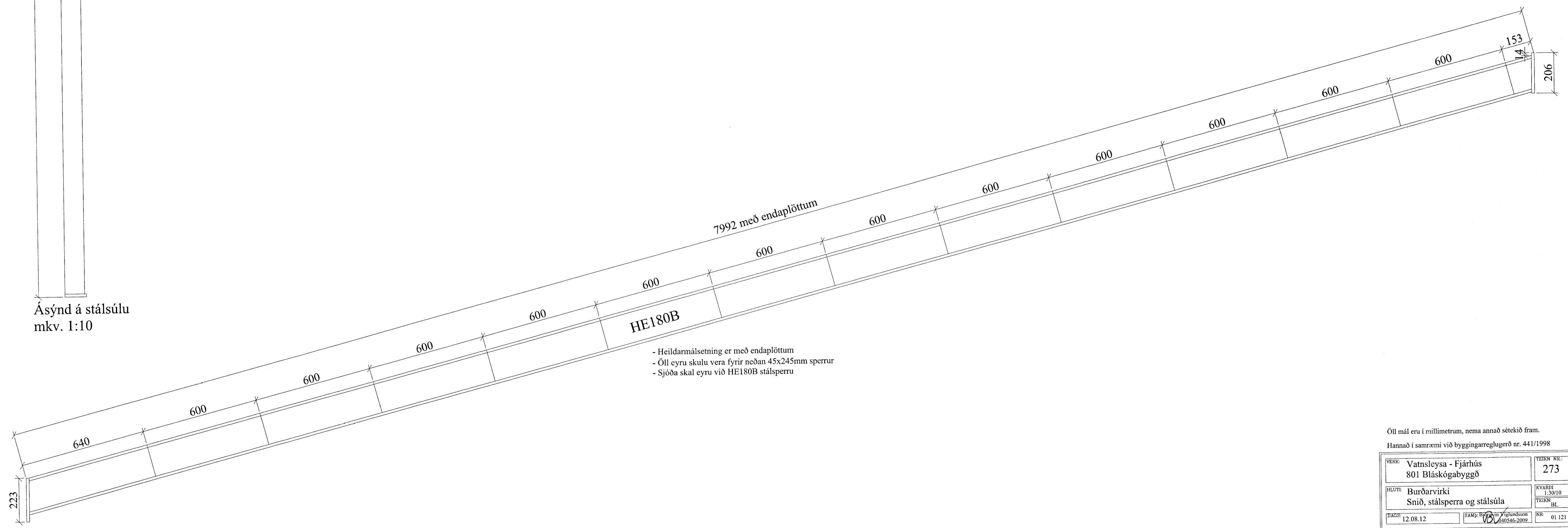
Ásýnd á HE-180B stálsperri mkv. 1:10
