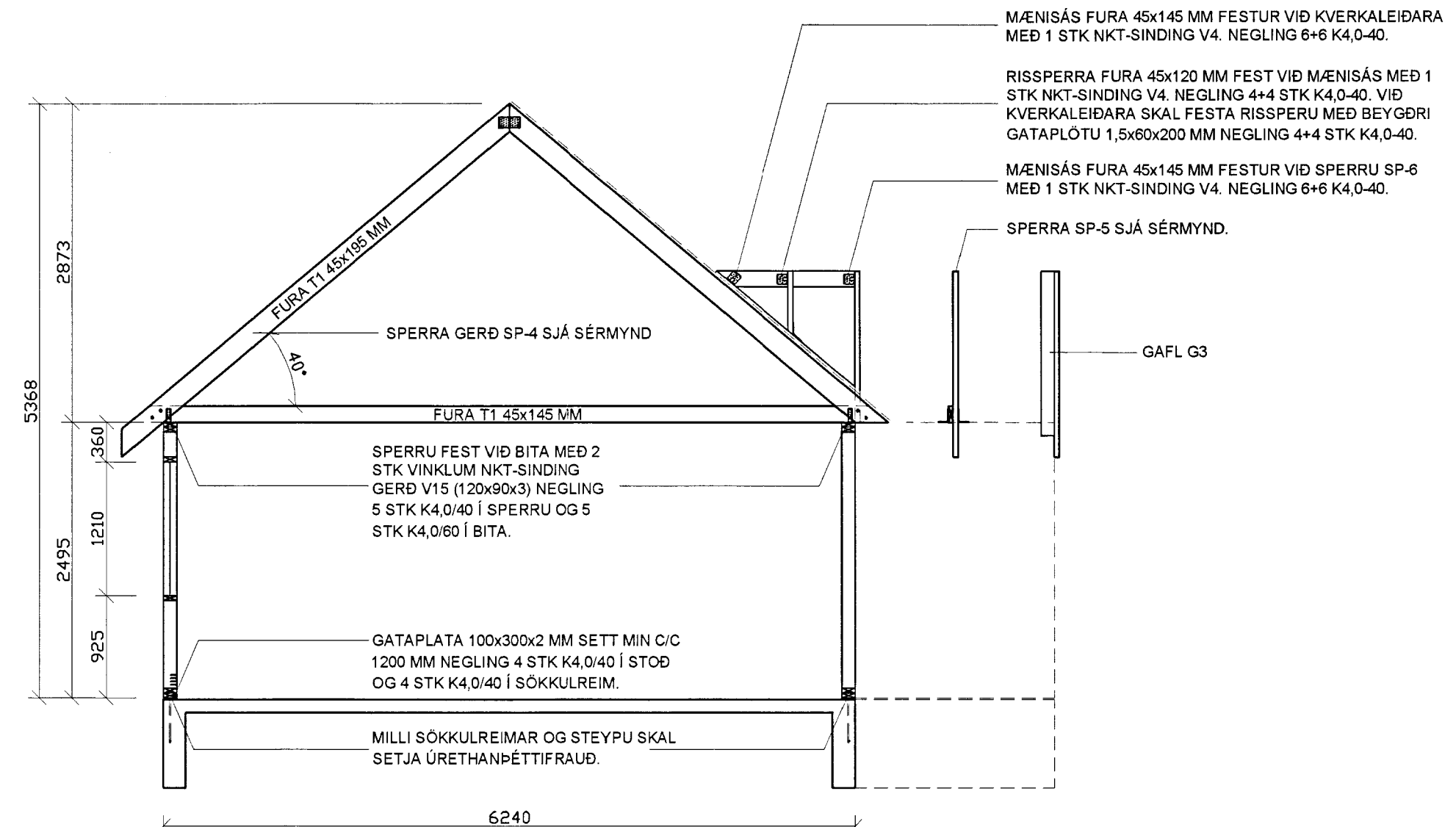
270 SNID 9 - 1:50
