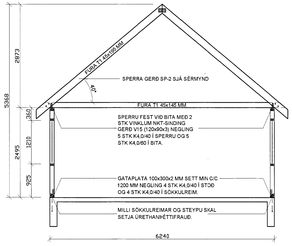
270 SNID 7 - 1:50
