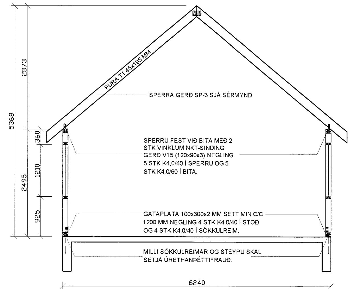
270 SNID 8 - 1:50
