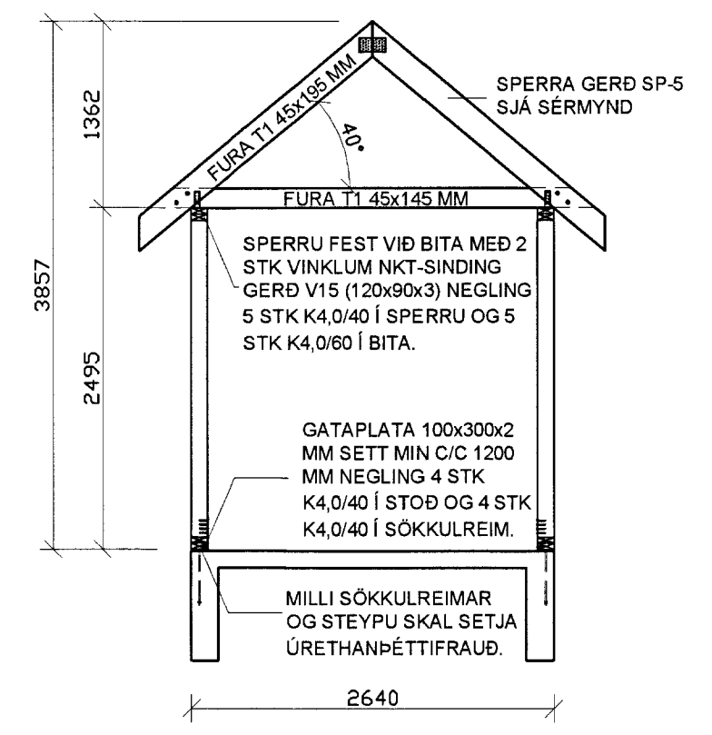
270 SNID 10 - 1:50
