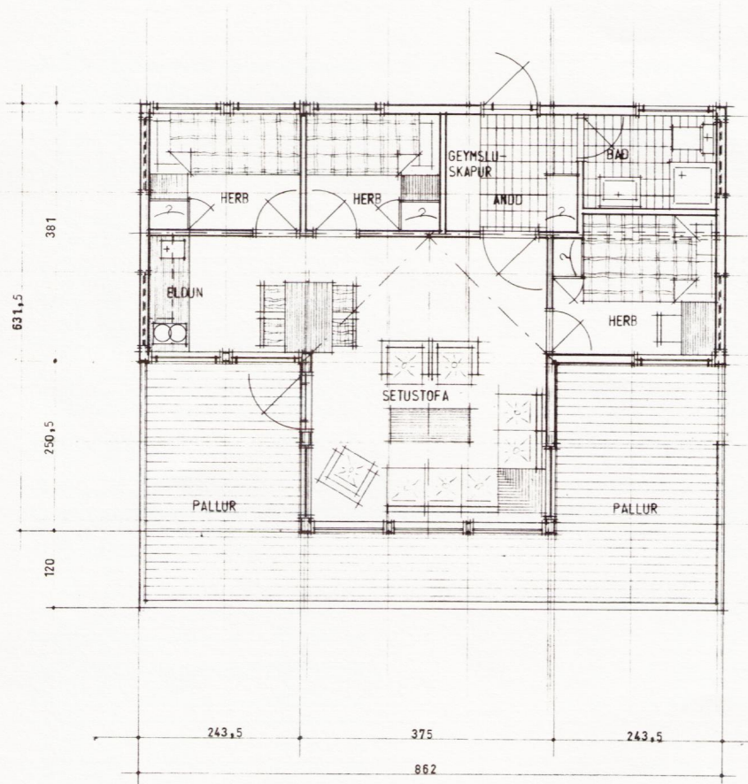
GRUNNMYND M 1:50
