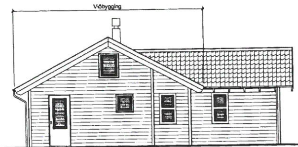
ÚTLIT NORDUR 1:100
