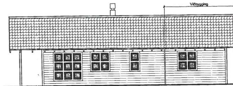
ÚTLIT AUSTUR 1:100
