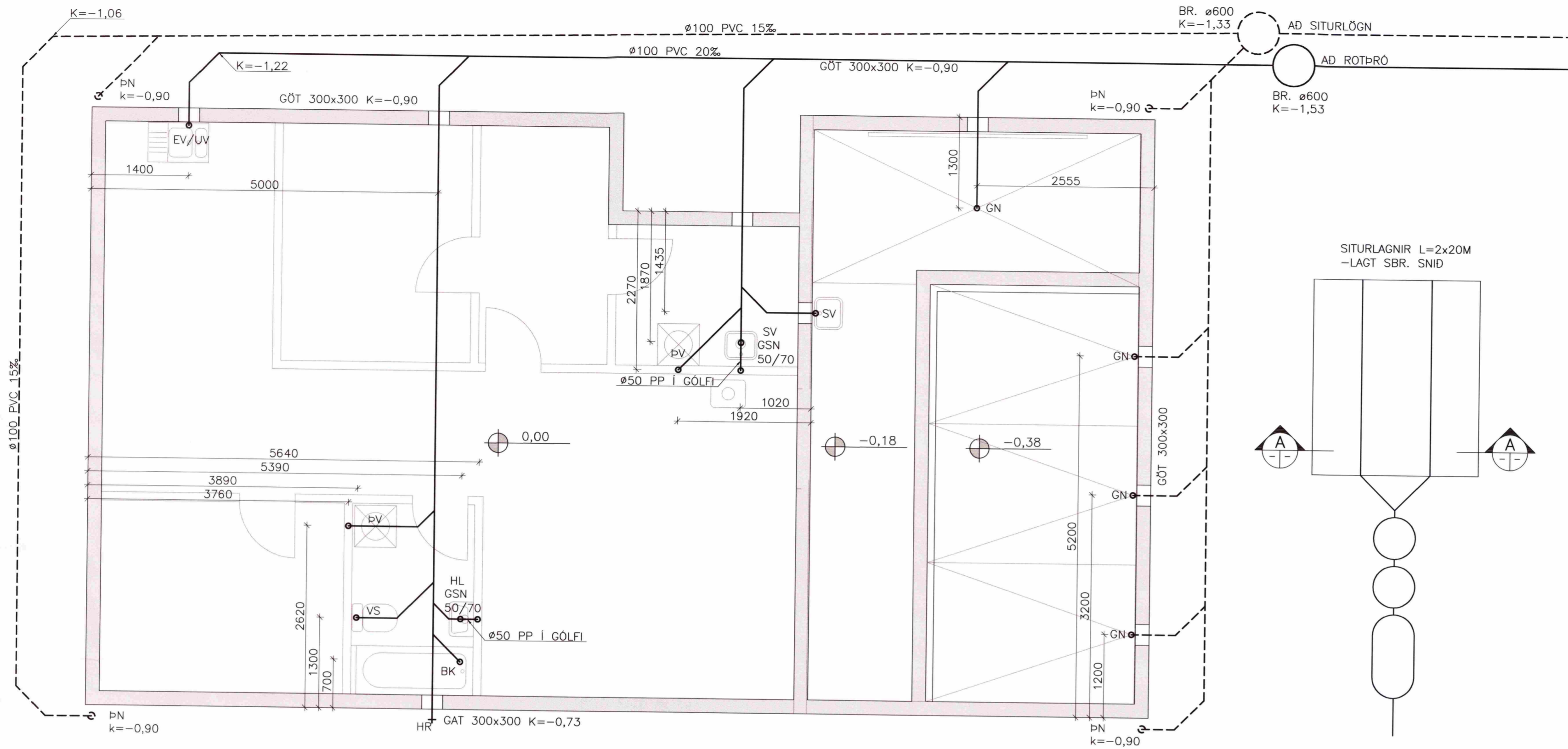
ROTÞRÓ, GRUNNMYND 1:50
