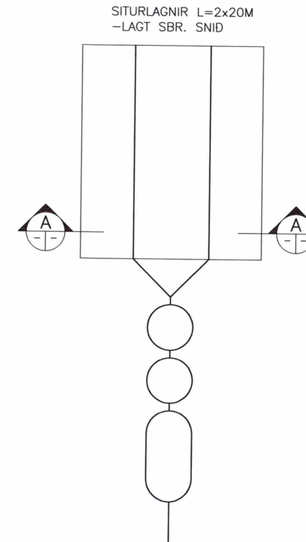
ROTÞRÓ, GRUNNMYND 1:50
