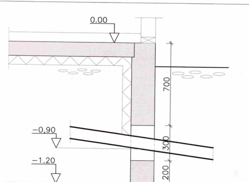
KÓTAR, SKÝRINGAR 1:20
