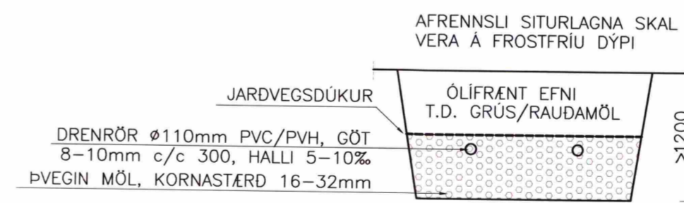
SITURLÖGN, SNID A-A 1:50
