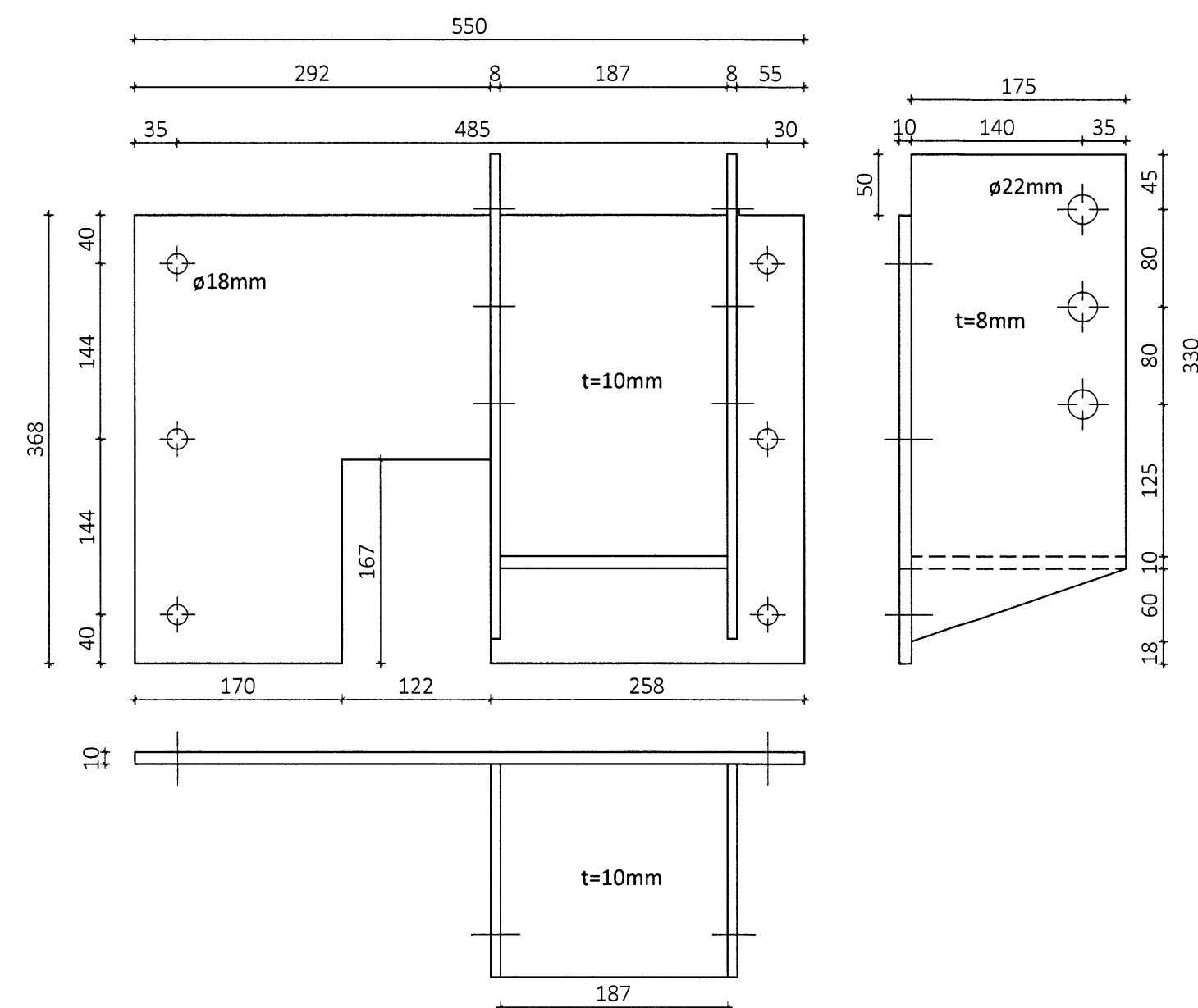
Stálfesting SF2 Mkv. 1:5 Samtals 1 stk + 1 stk speglað
