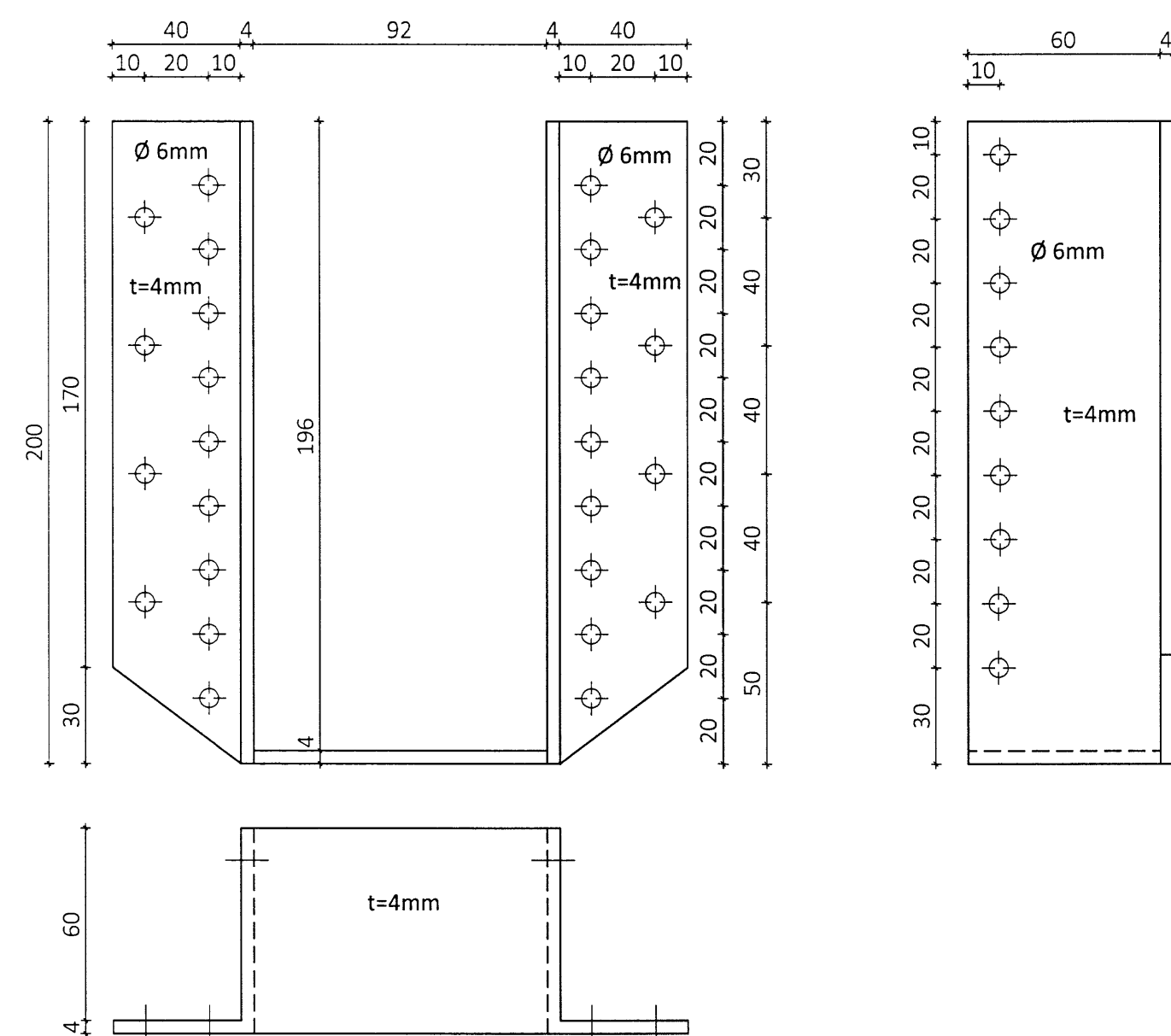
Stálfesting BS1 90x200 Mkv. 1:2 Samtals: 40 stk
