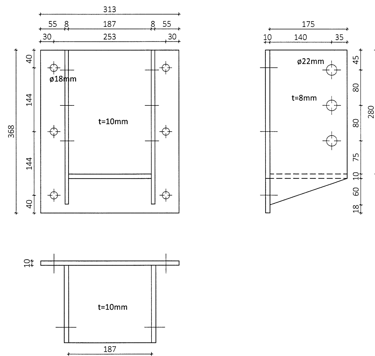
Stálfesting SF1 Mkv. 1:5 Samtals 18 stk
