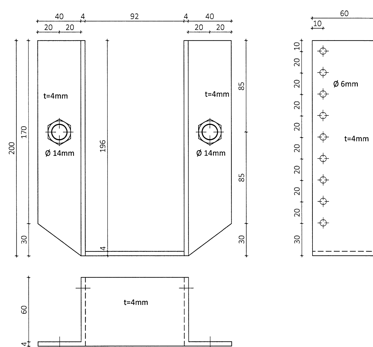
Stálfesting BS2 90x200B Mkv. 1:2 Samtals: 4 stk
