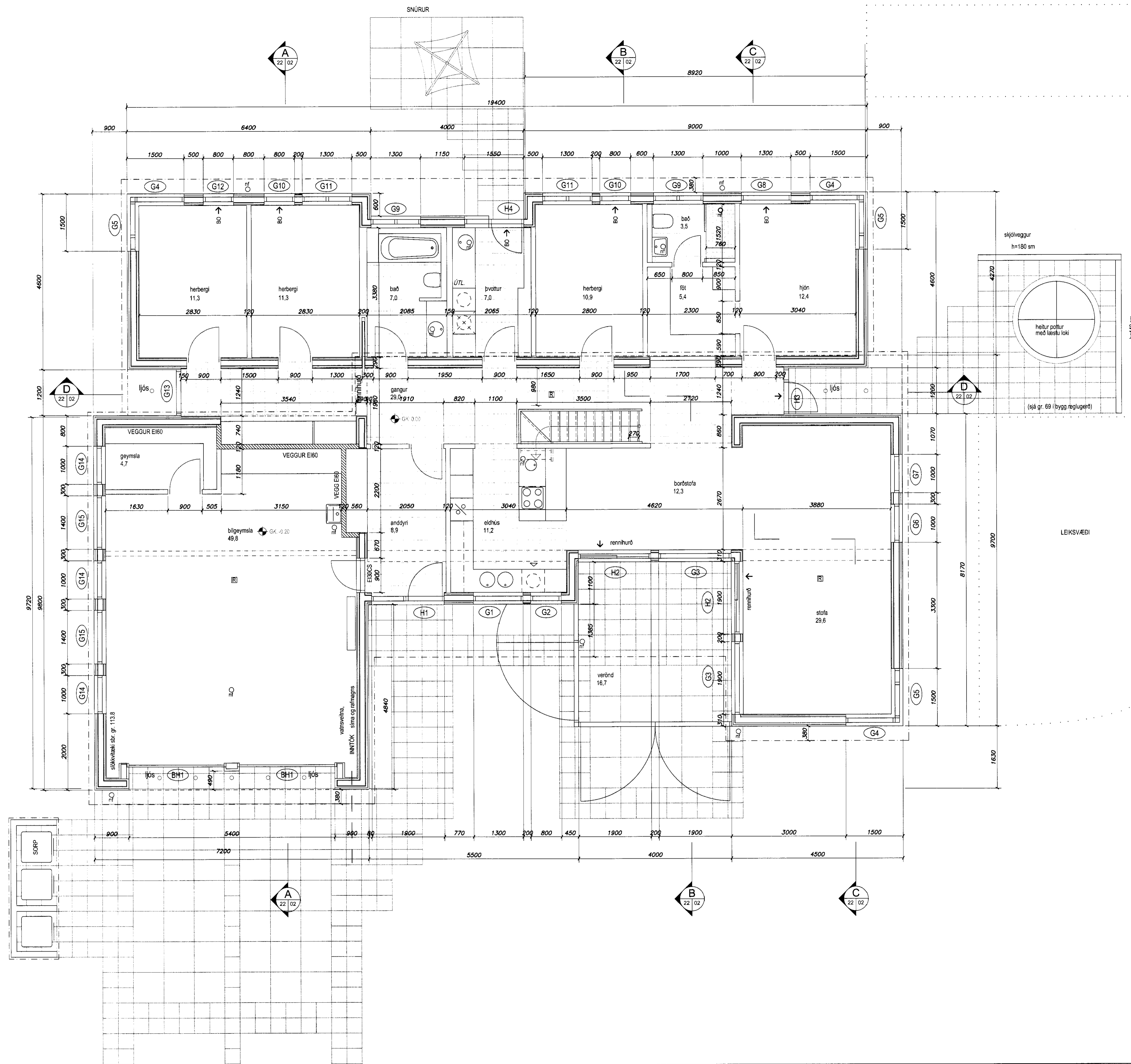
GRUNNMYND 1:50
