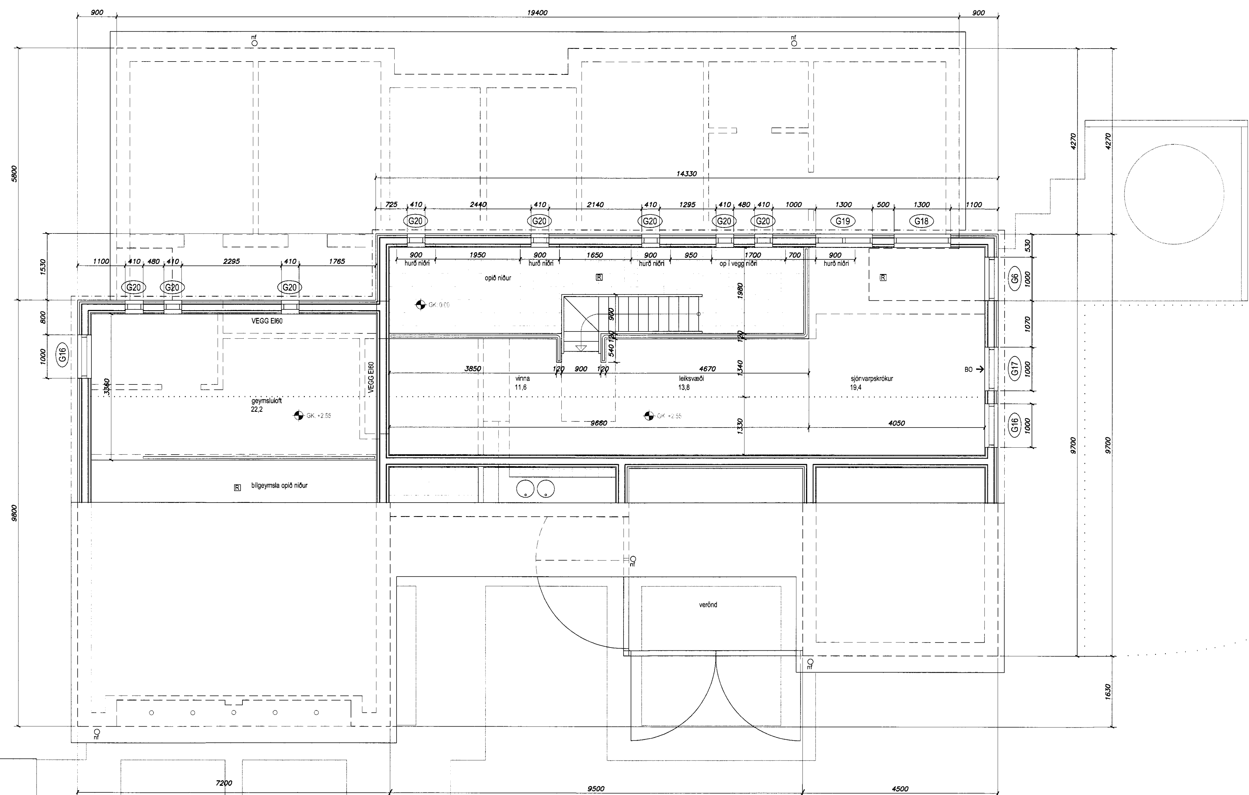
GRUNNMYND, MILLIPALUR 1:50
