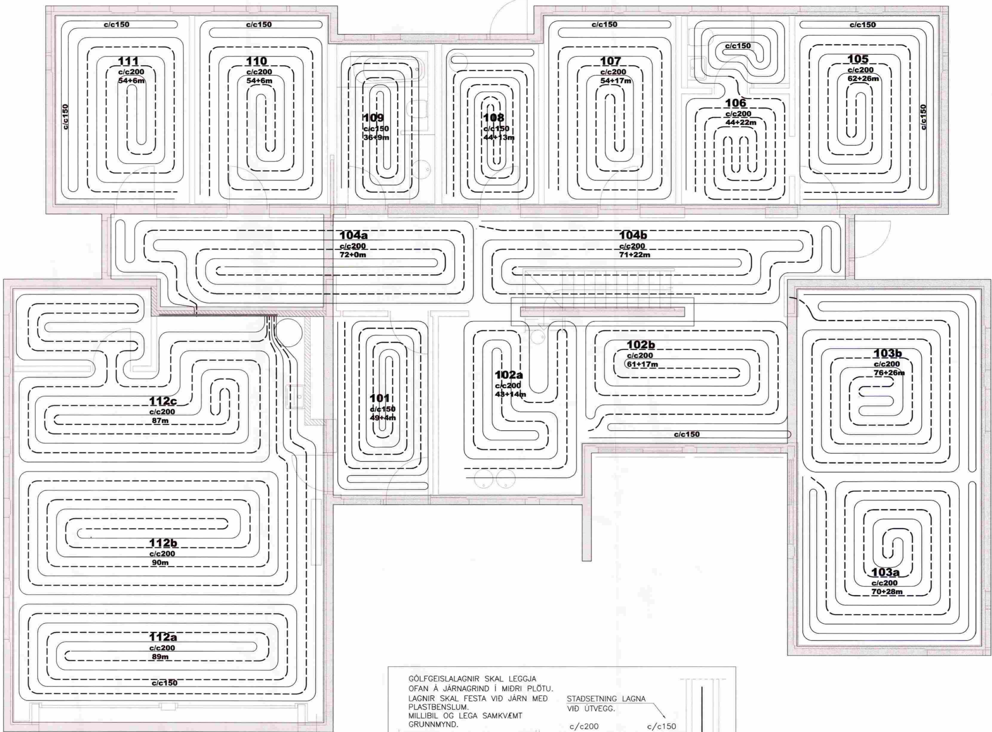
GÖLFHITALAGNIR – GRUNNMYND 1:50
