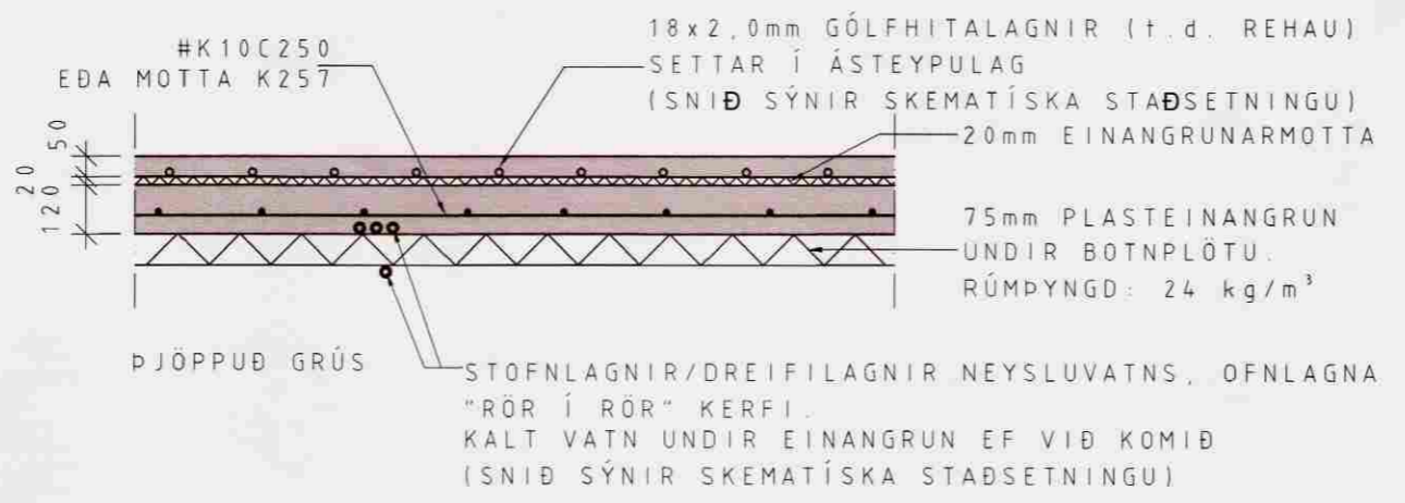
ALMENNT SNÍÐ Í BOTNPLÖTU 1:20
