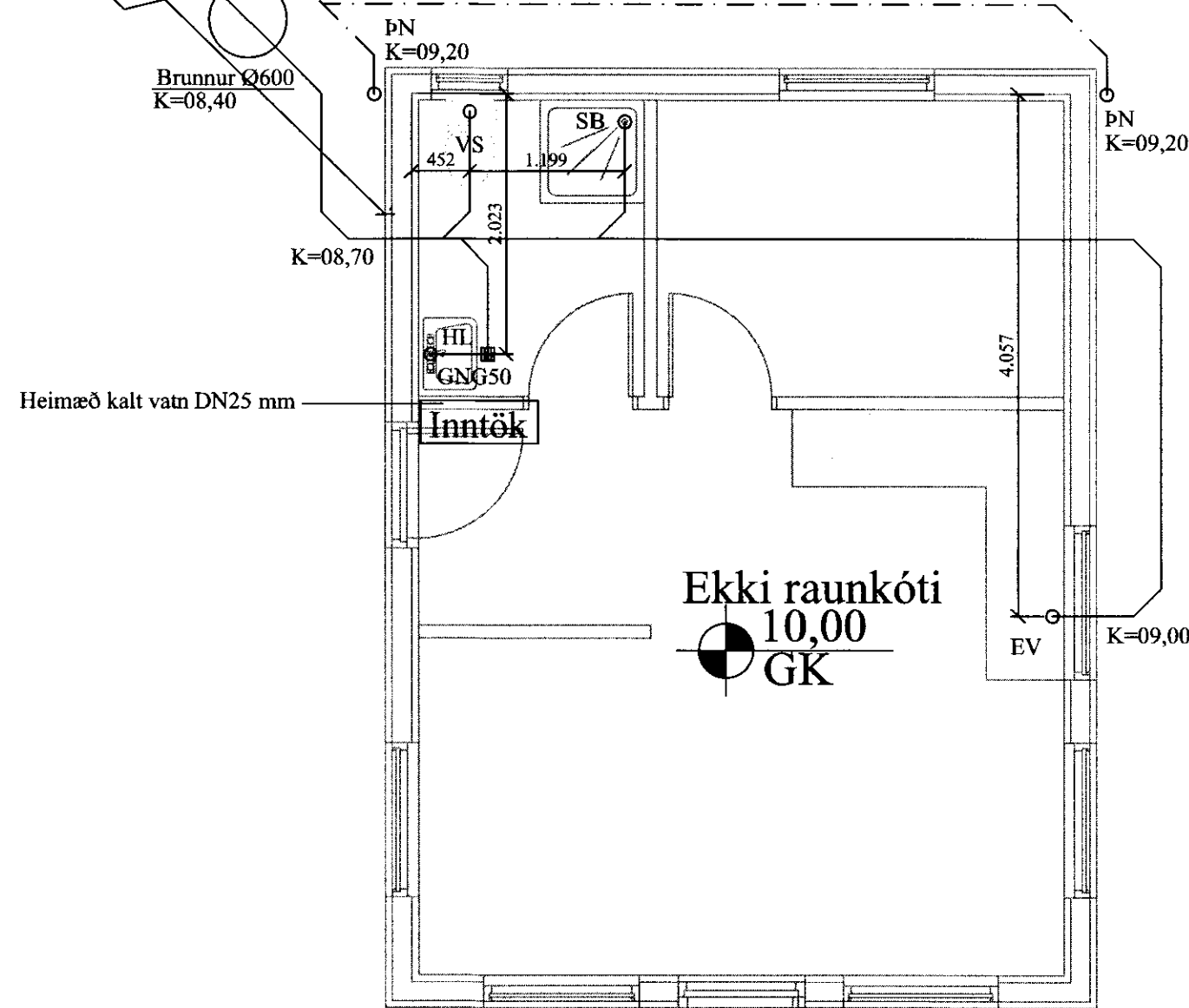
Grunnmynd frárennslislagna mkv. 1:50
