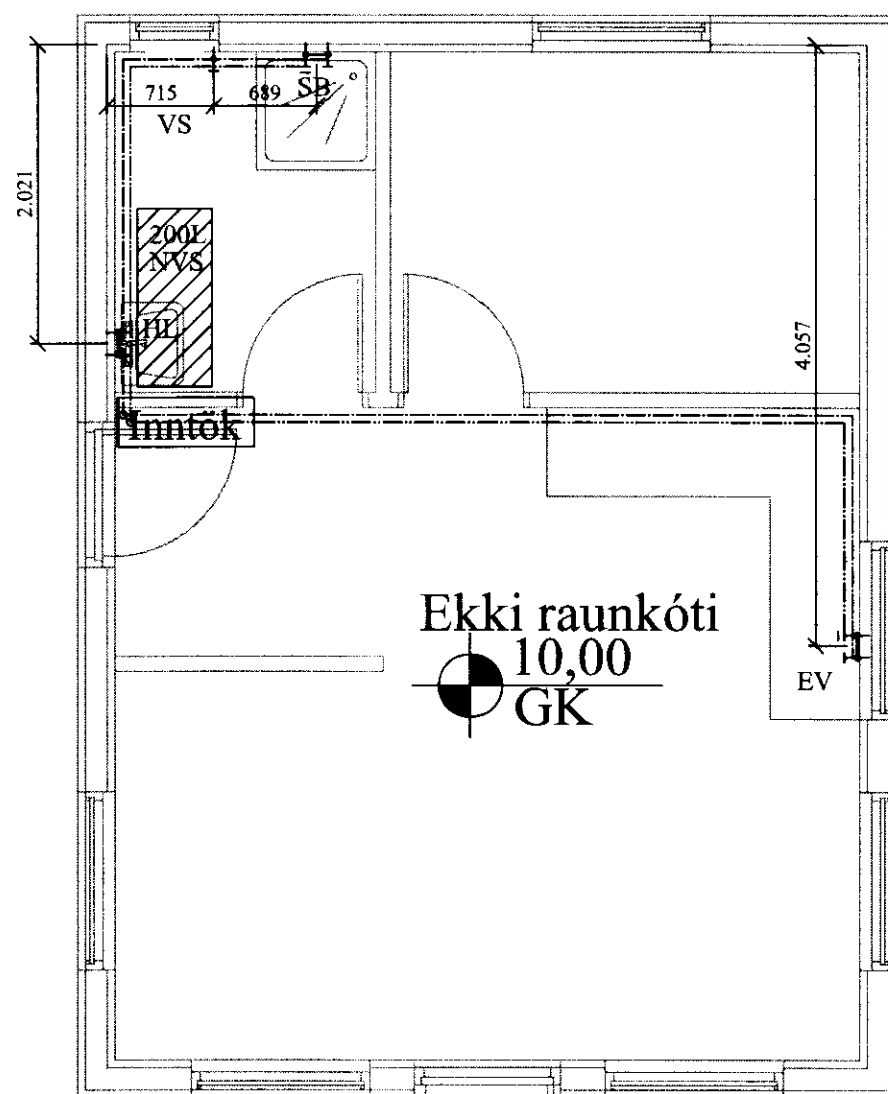
Grunnmynd neysluvatnslagna mkv. 1:50
