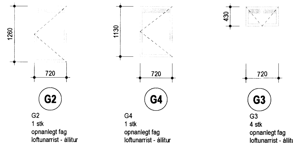
3 ÚTLIT - GLUGGAR Í VEGGLÆÐINGU 1:50
