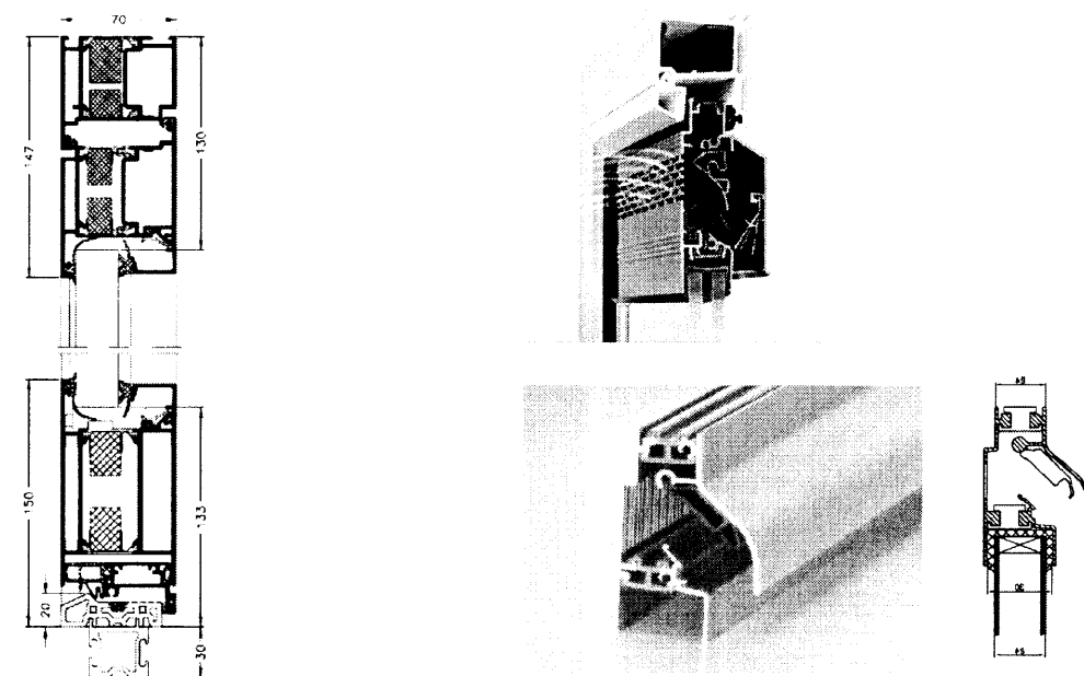
5 DEILI - ÁLHURÐ 1:5
