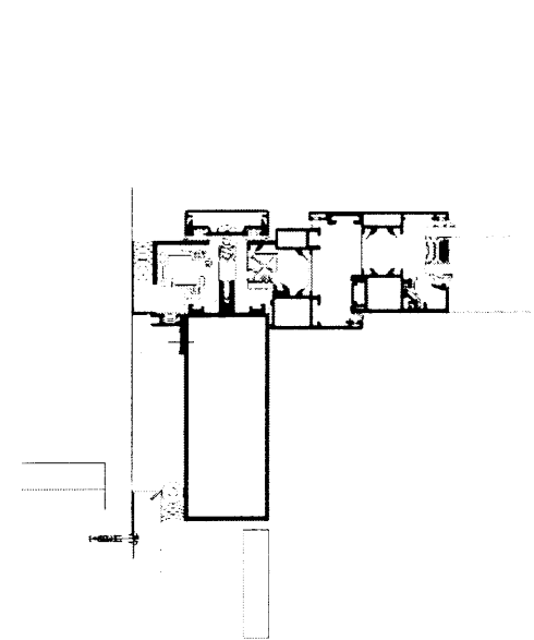
3 HURÐ H1 - INNGANGUR 1:50
