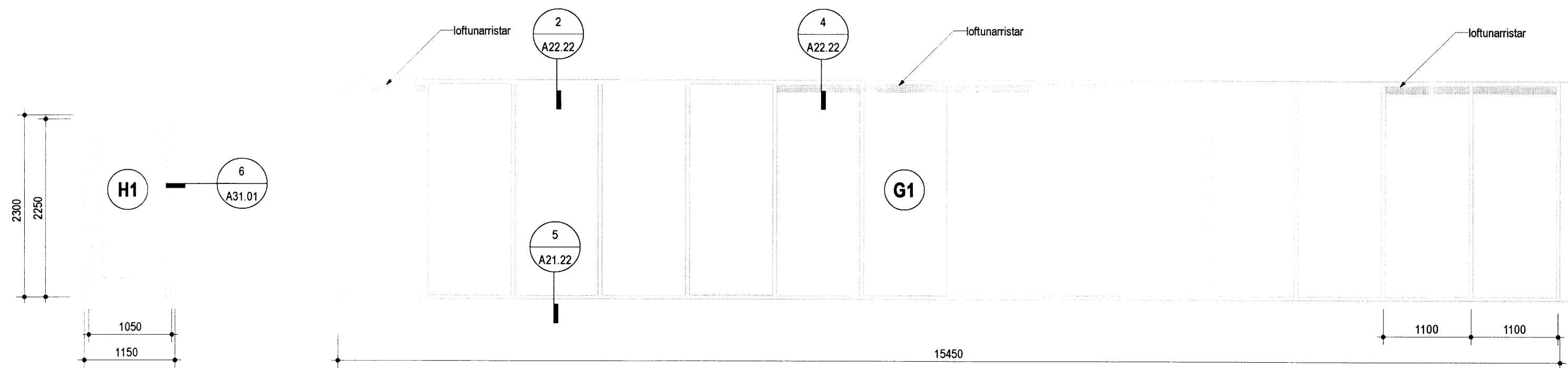
3 HURÐ H1 - INNGANGUR 1:50
