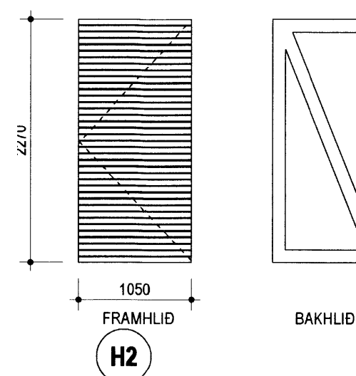
4 DEILI - LOFTUNARRISTAR 1:5
