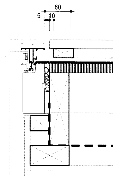
7 DEILI - VALMÖGULEIKI; GLUGGAKARMUR INNAR Í VEGGLÍFI 1:5
