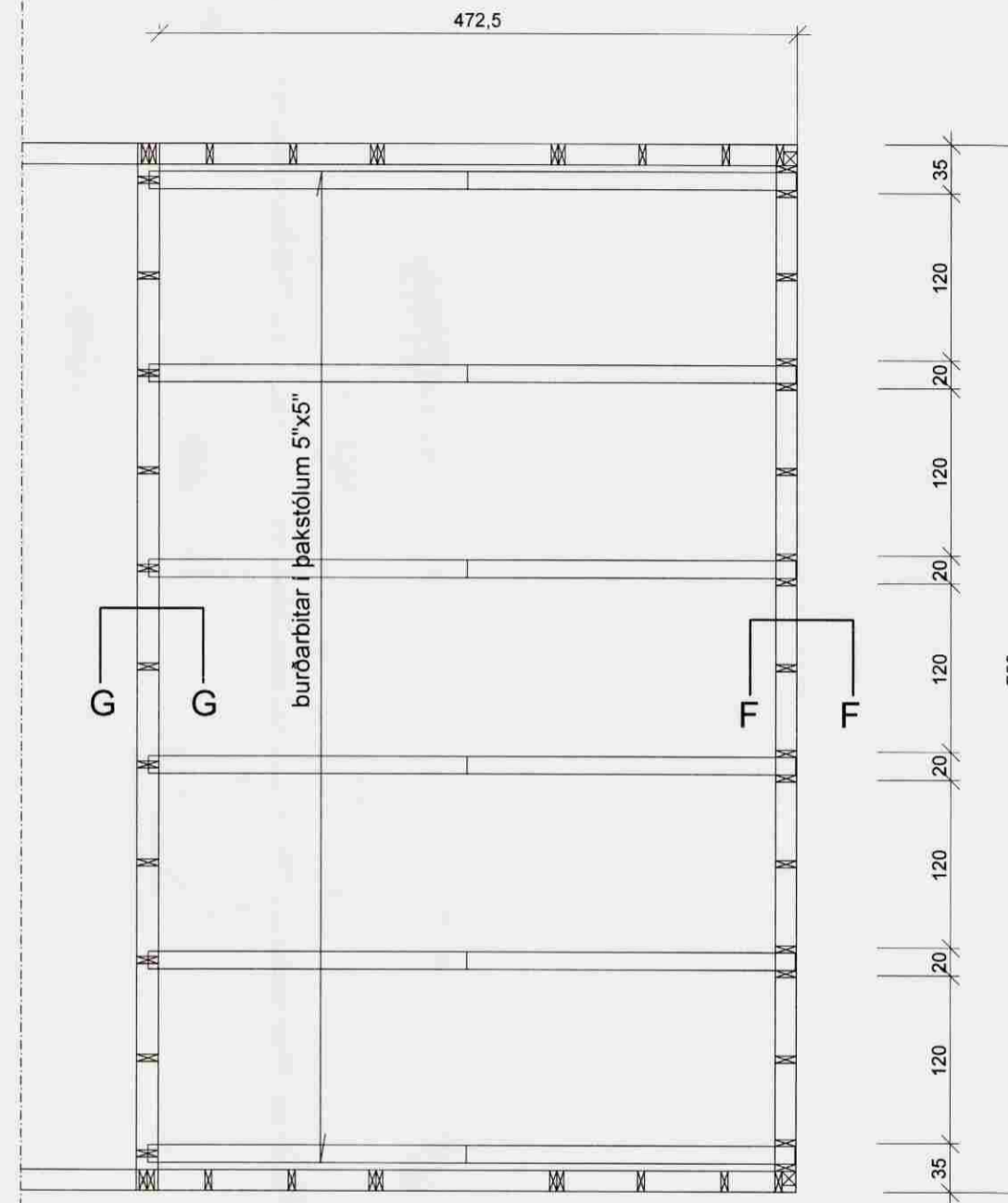
Grunnmynd 1:50, þakstólar - syðri endi
