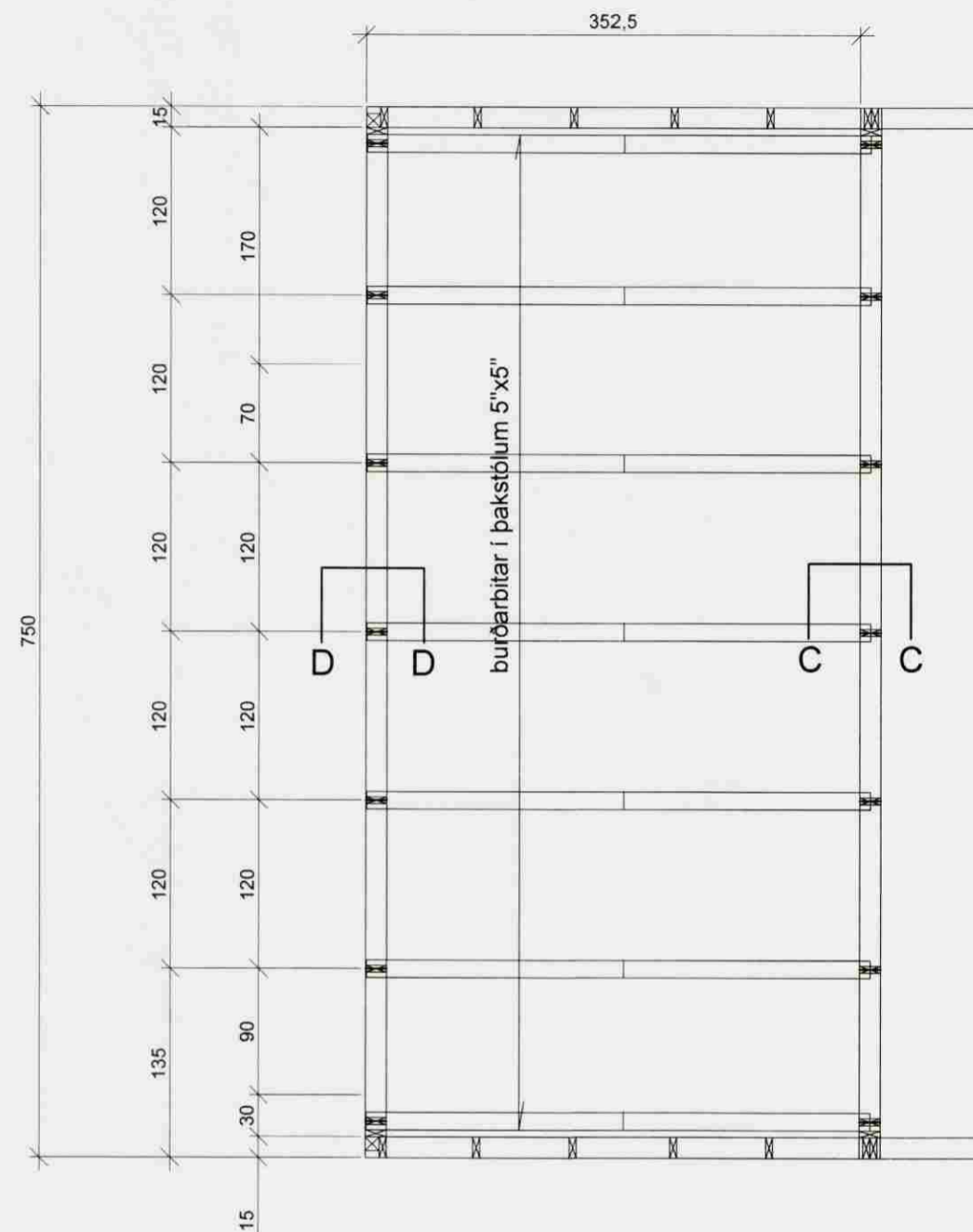
Grunnmynd 1:50, þakstólar - norður endi
