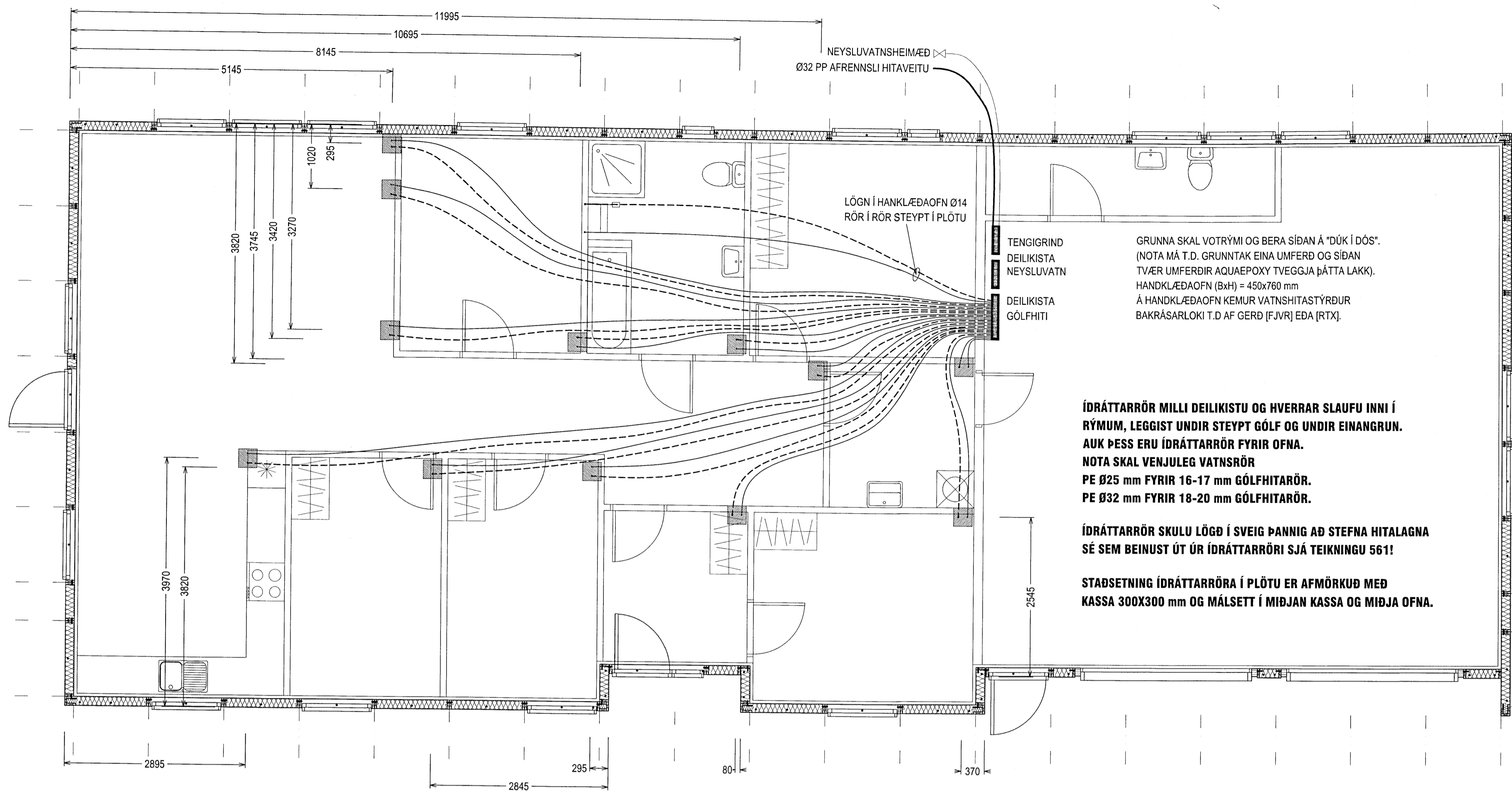
GRUNNMYND IDRÁTTARRÖRA FYRIR GÓLFHITA OG OFNA Mkv. 1:50
