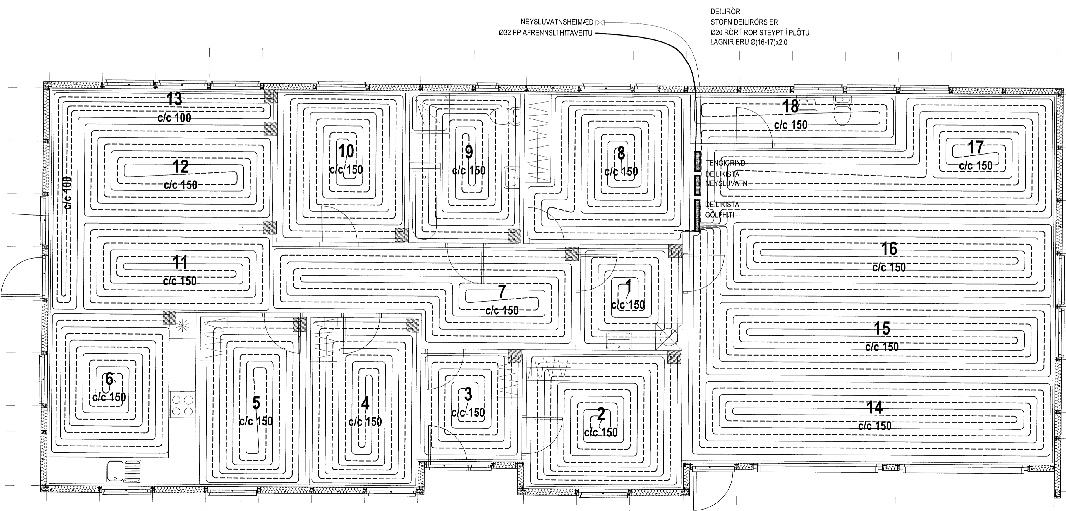
GRUNNMYND IDRÁTTARRÖRA FYRIR GÓLFHITA OG OFNA Mkv. 1:50
