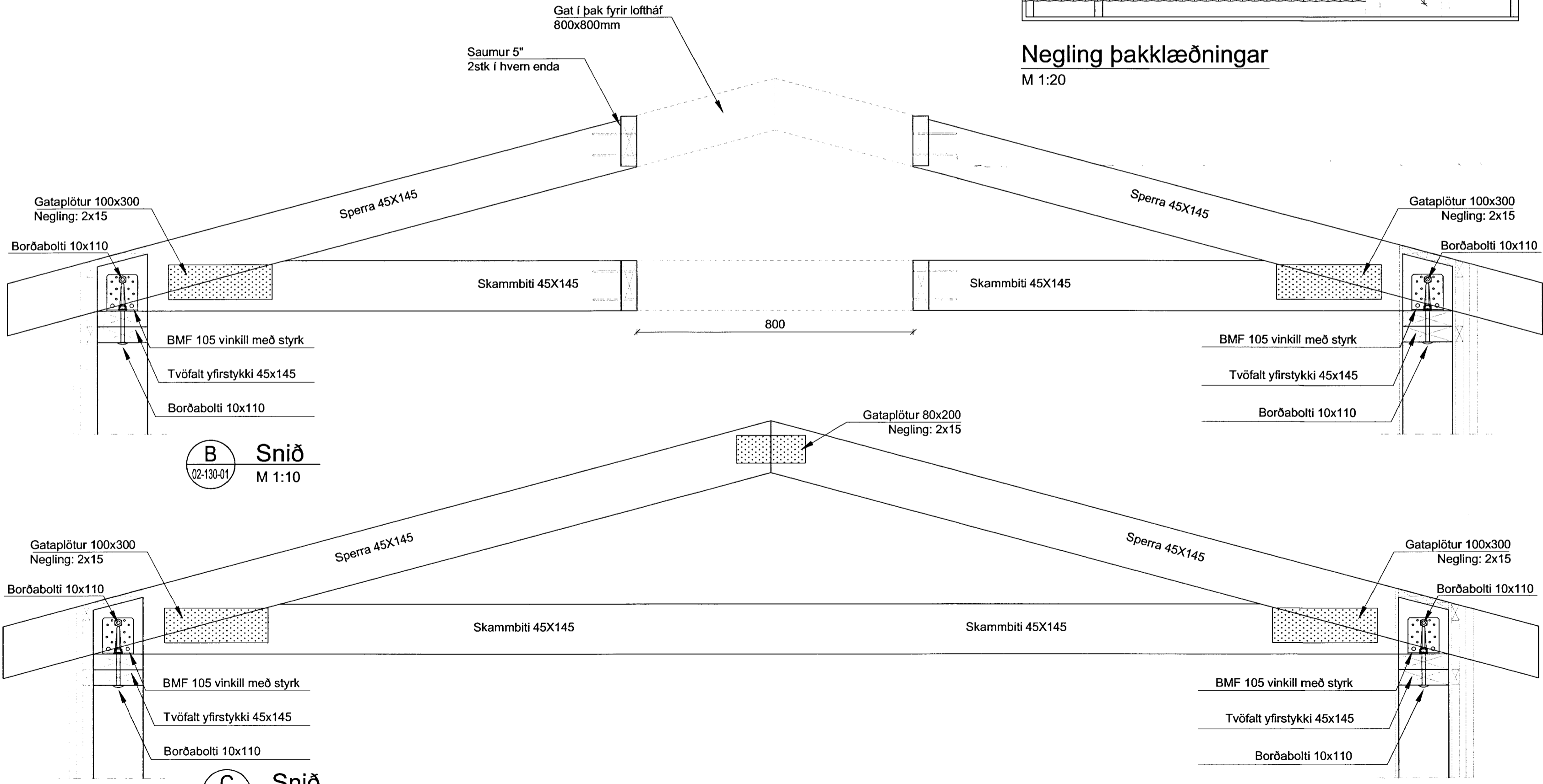
C Snið M 1:10
