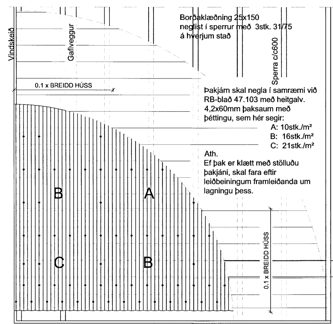
Negling þakklæðingar M 1:20
