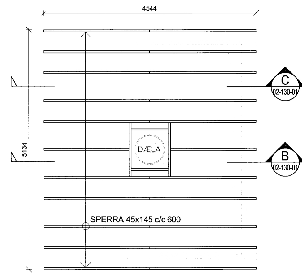
Paksperruplan M 1:50
