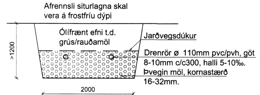
AA Snið M 1:50
