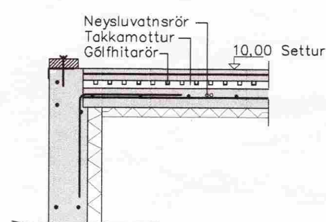
Lagnir í gólf 1:20
