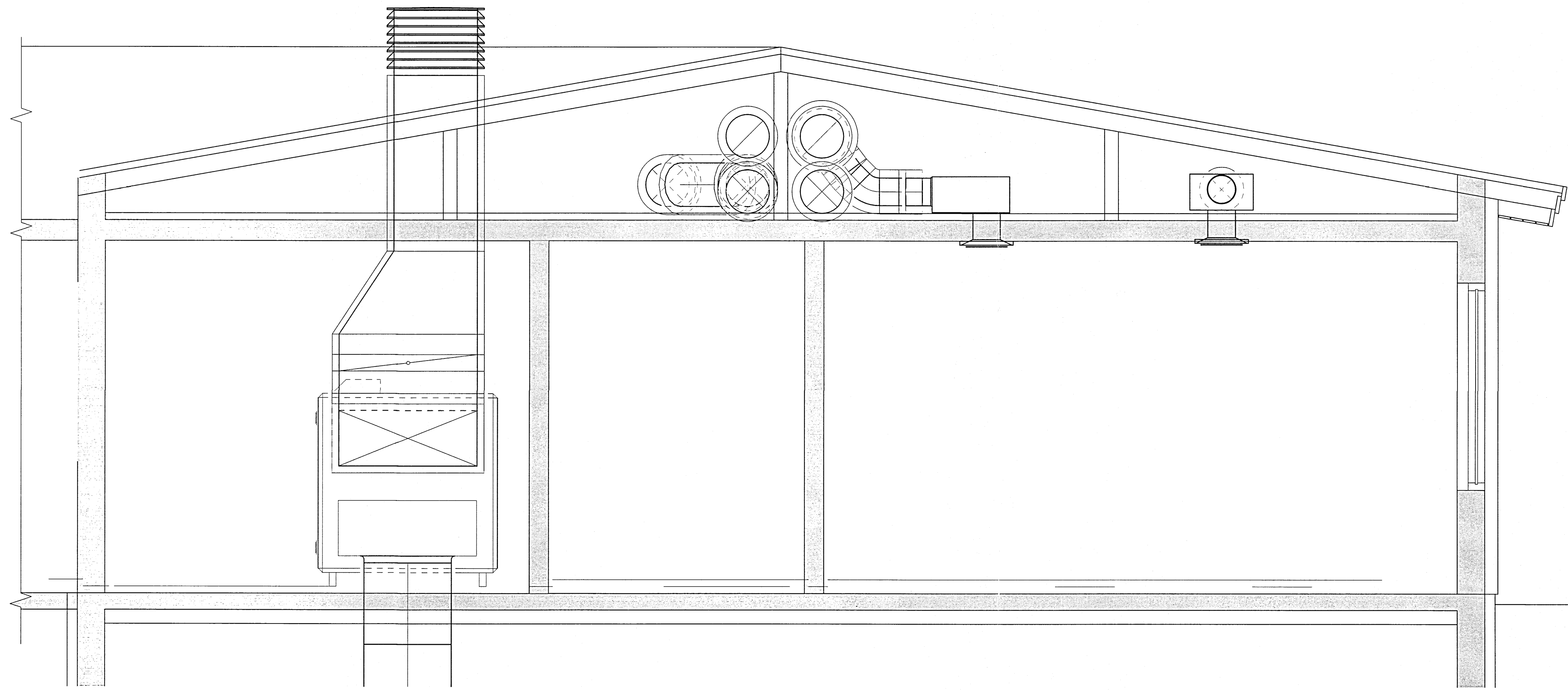
SNID B-B - Mkv.: 1:20
