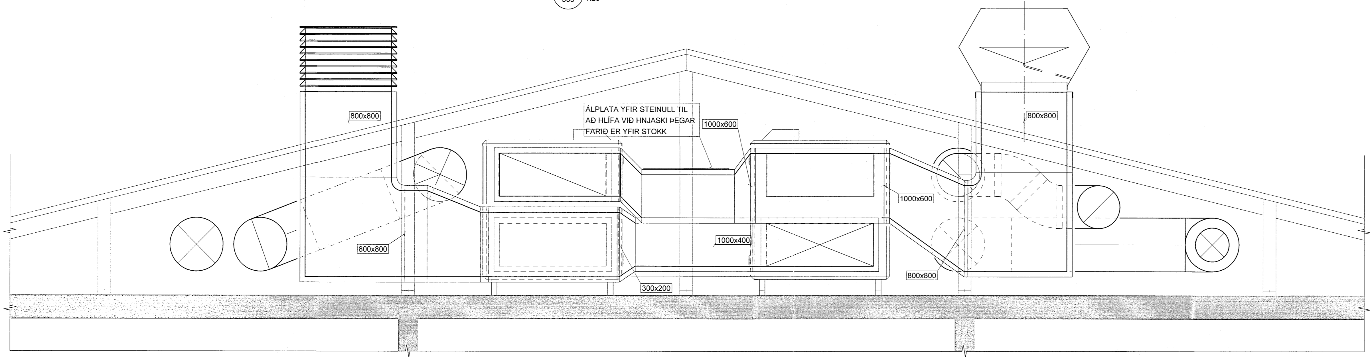
E SNÍÐ 503 1:20
