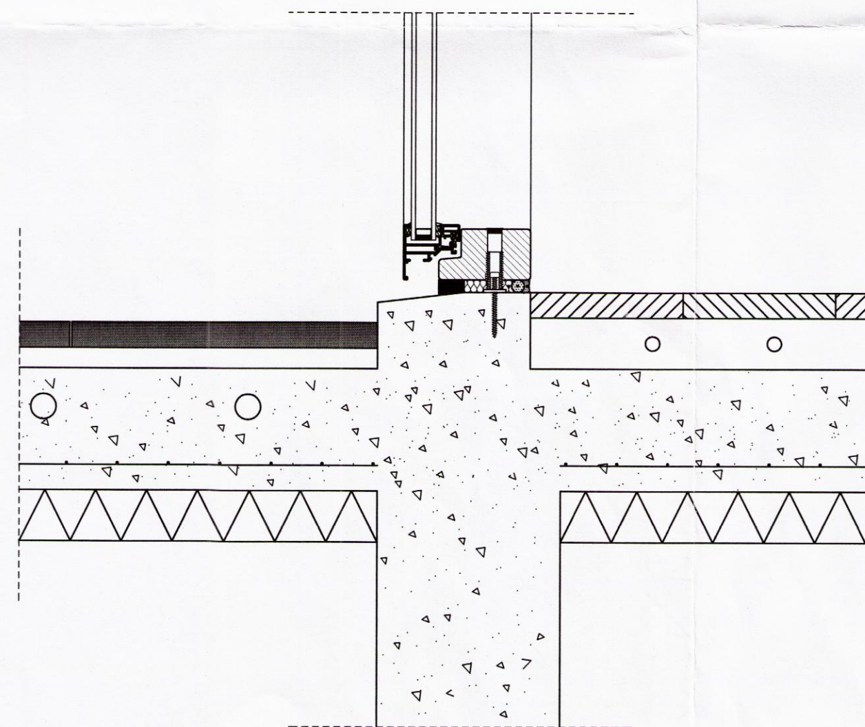
Frágangur glugga við gólf - lóðrétt deili 1:5
