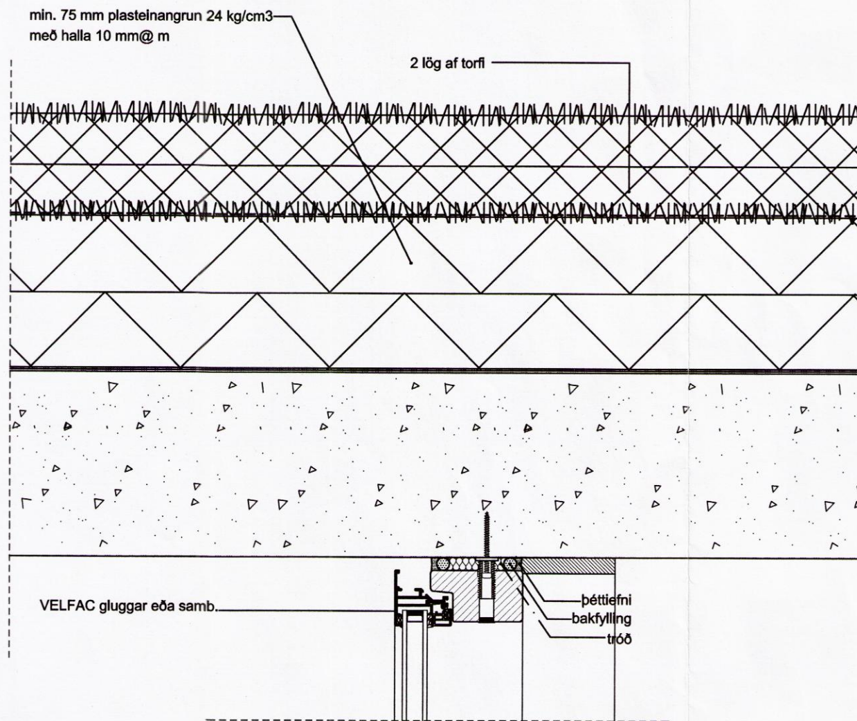
Frágangur glugga við þak - lóðrétt deili 1:5
