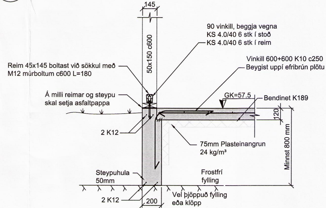
A Snið B-010 Mkv. 1:20
