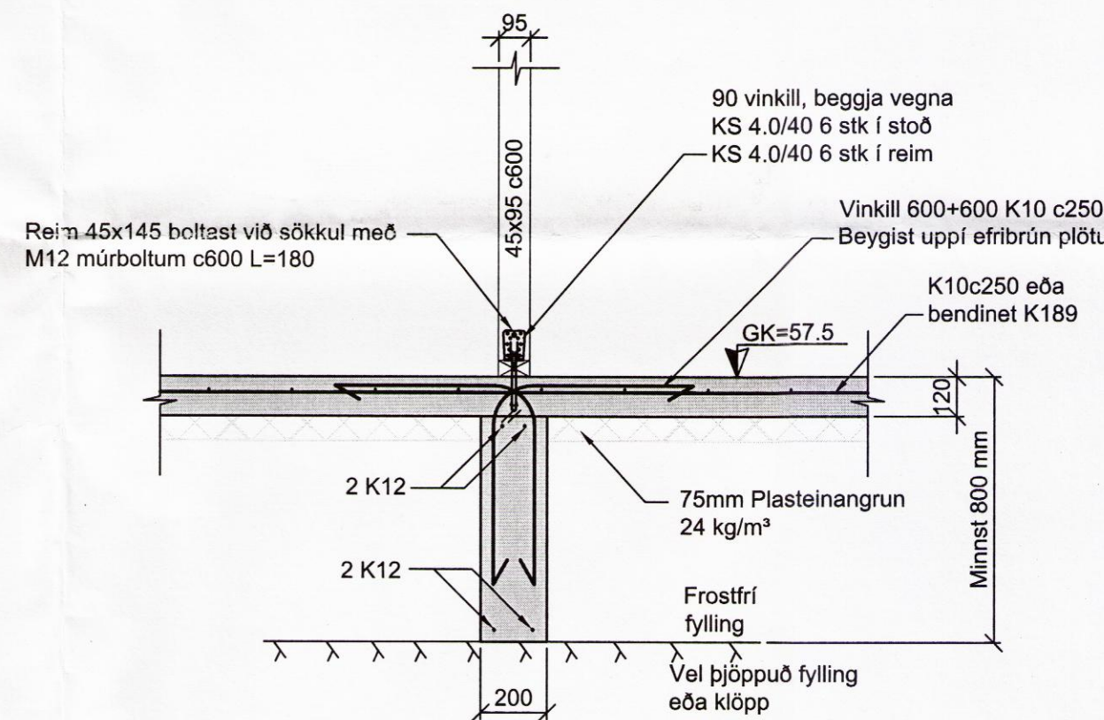
B Snið B-010 Mkv. 1:20
