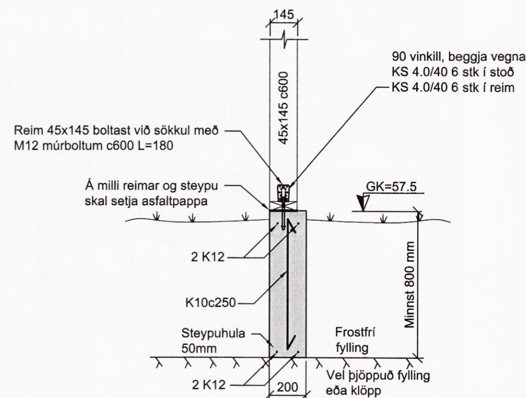
C Snið B-010 Mkv. 1:20
