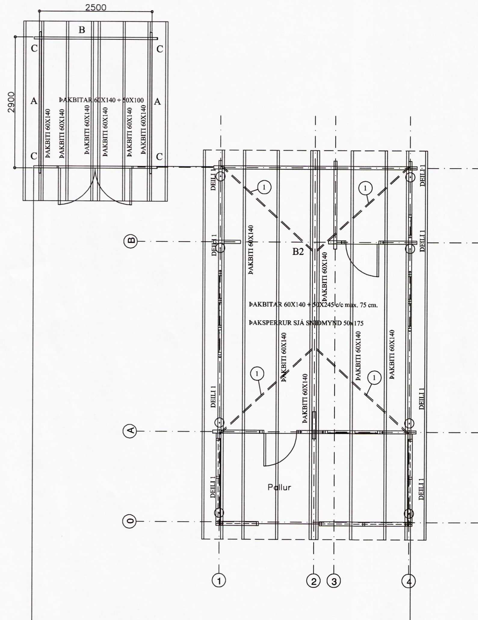
Grunnmynd þak
