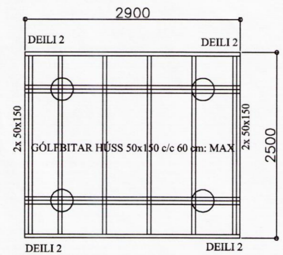
Grunnmynd gólfbitar
