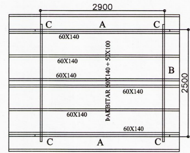
Grunnmynd þak
