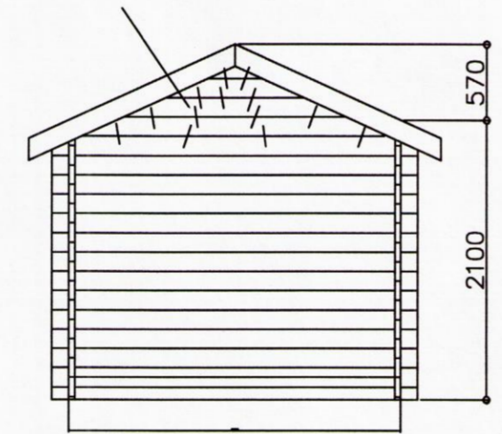
Hliðarmynd gabl festing skásagaðra bjálka
