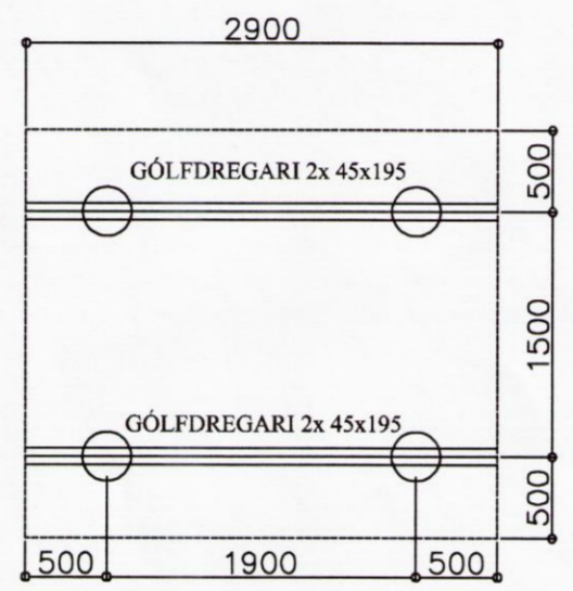
Grunnmynd dregarar
