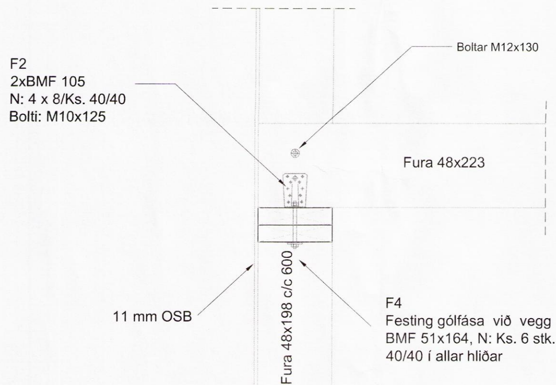
E Snið í útvegg Mkv. 1:10
