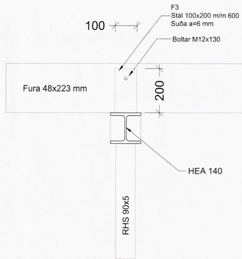
D Stálbitar og bitar í þakvirki Mkv. 1:10
