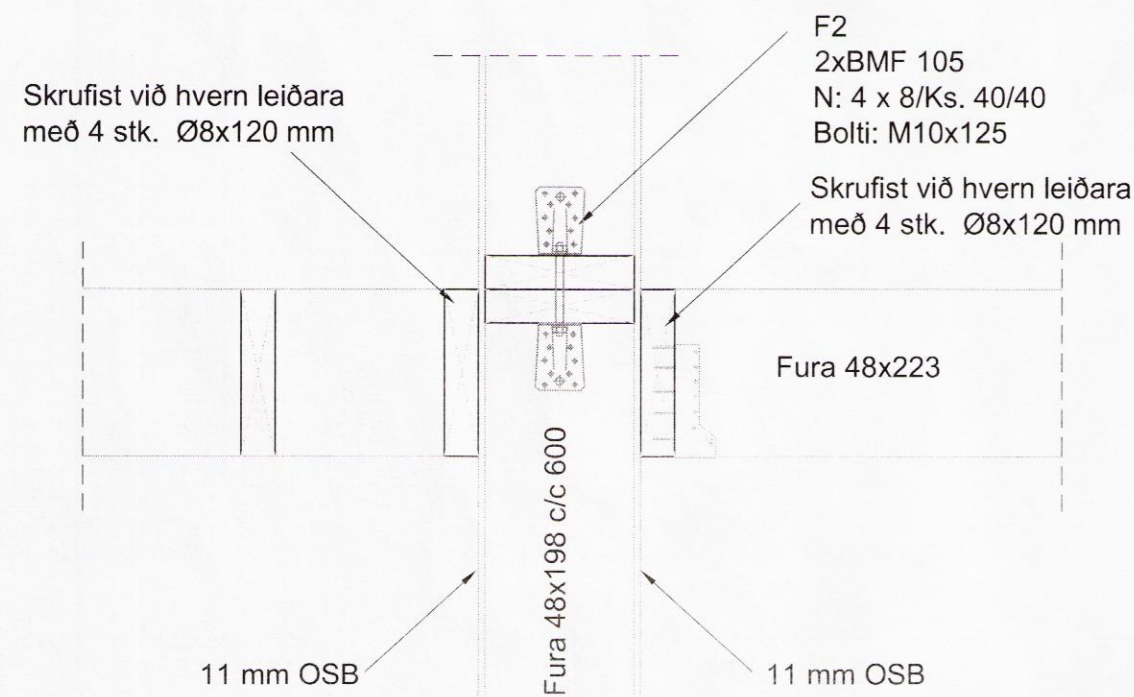
G Snið í vegg og þakvirki Mkv. 1:10
