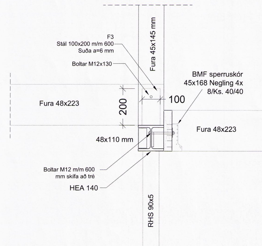
I Stálbitar og bitar í lofti Mkv. 1:10
