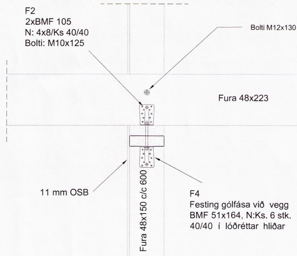
F Snið í millivegg og þakvirki Mkv. 1:10
