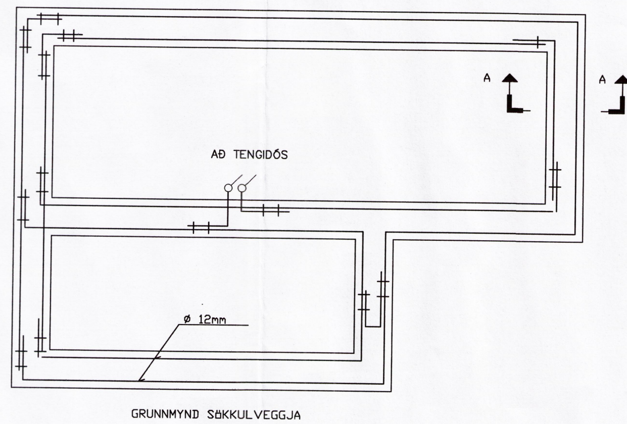
GRUNNMYND SÖKKULVEGGJA
