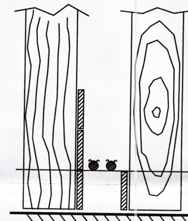
SNID A - A Í SÖKKULVEGG SÝND ERU 2 NEDSTU STEYPU- STYRKJARJÄRN Í STEYPUMÓTI OFAN Á NEDSTU MÖTAMRUM
