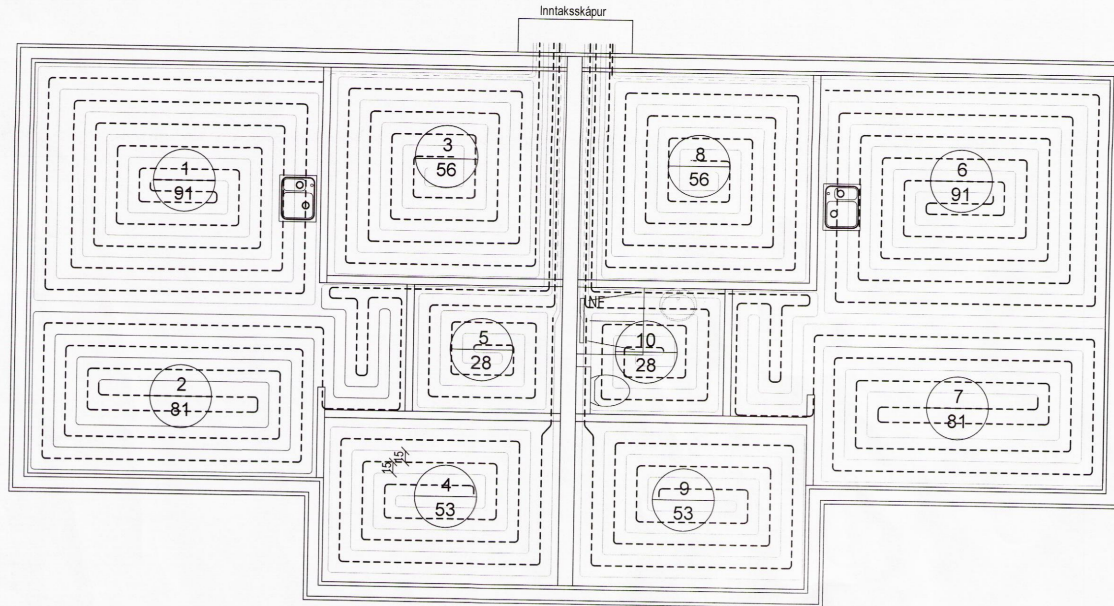
GÓLFHITI, GRUNNMYND 1:50
