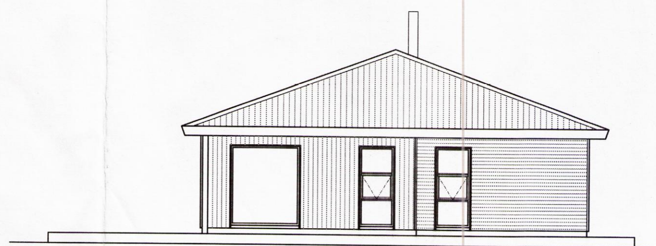
ÚTLIT AUSTUR ÍBÚÐARHÚS
